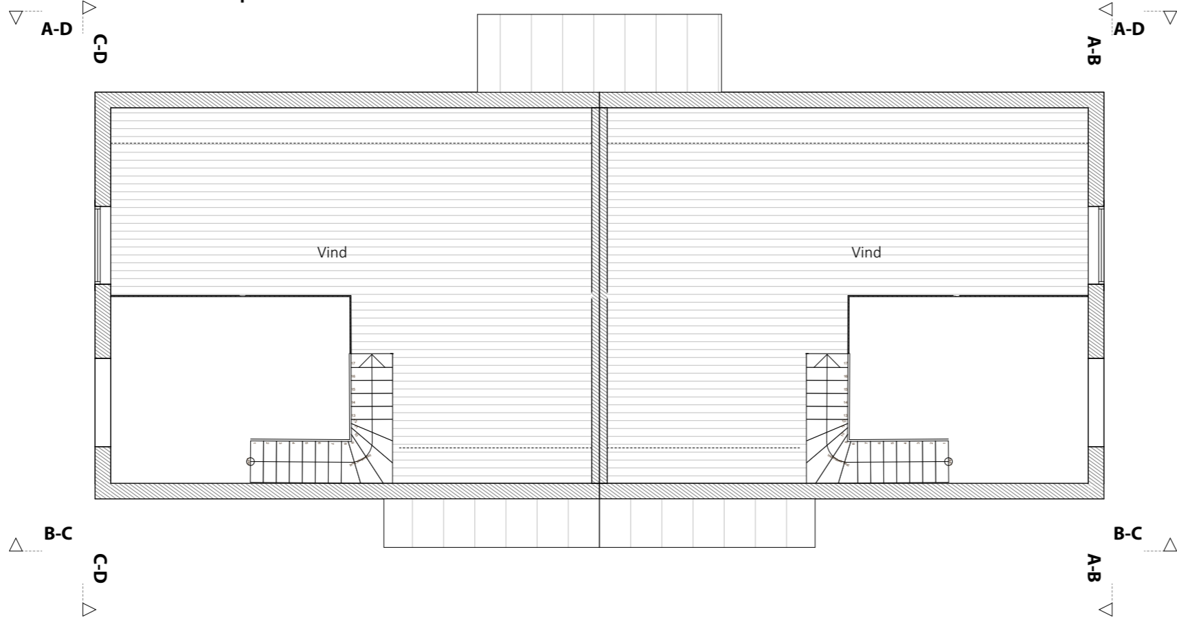
Vindsplan
