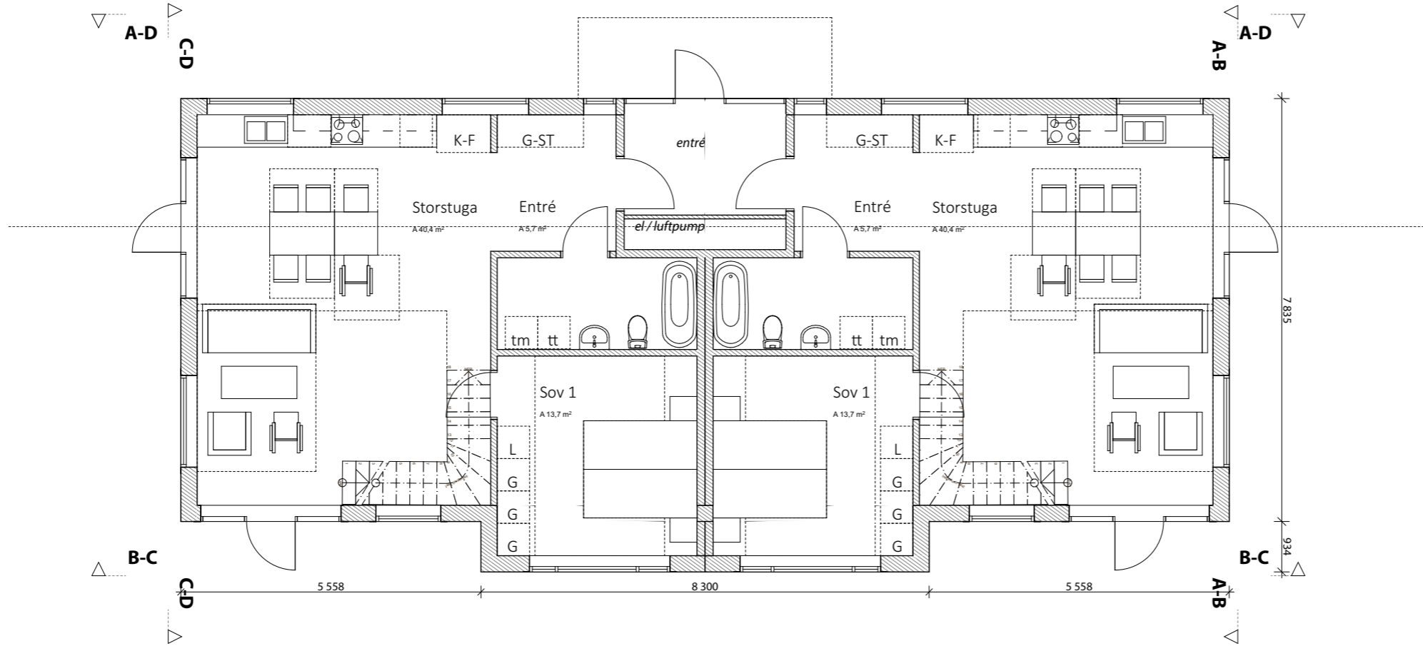
Bostadsplan
