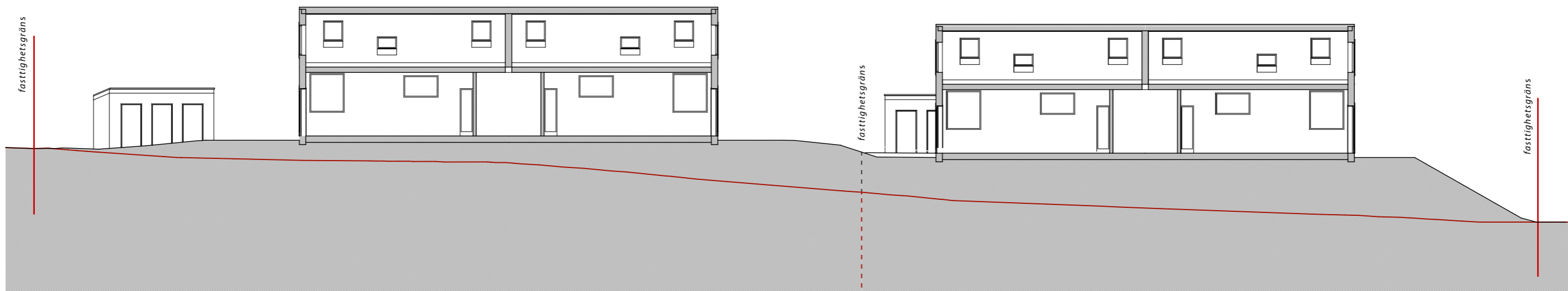
Kvarterssektion
