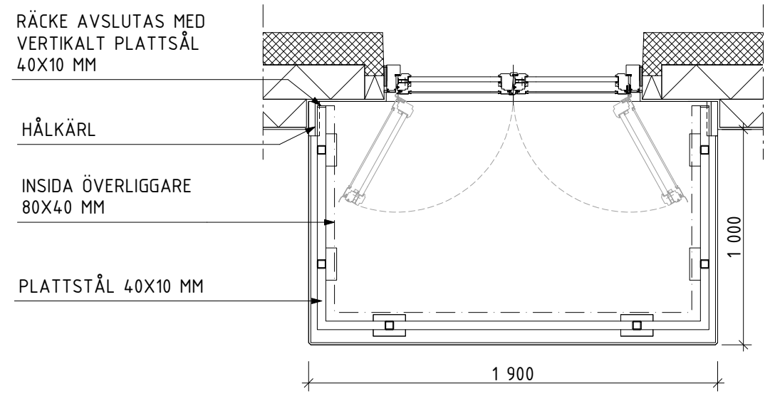
PLANUTSNITT
