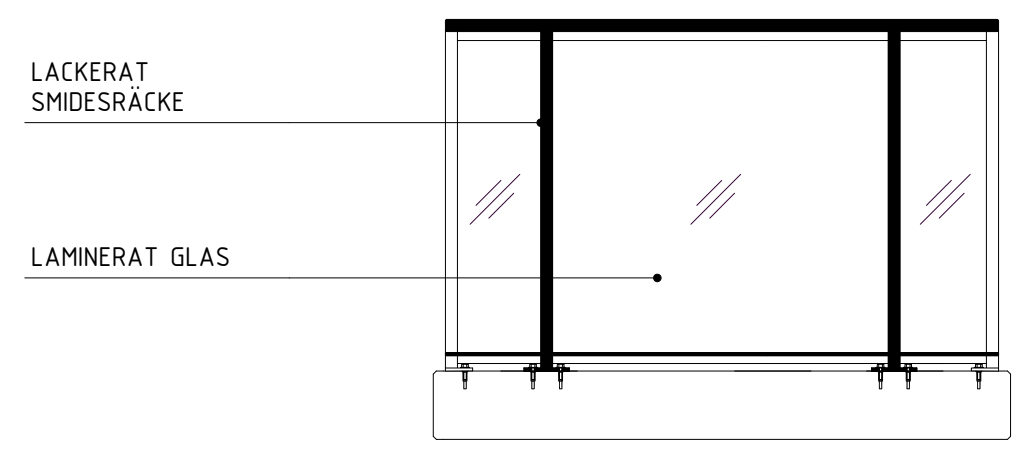
ELEVATION
