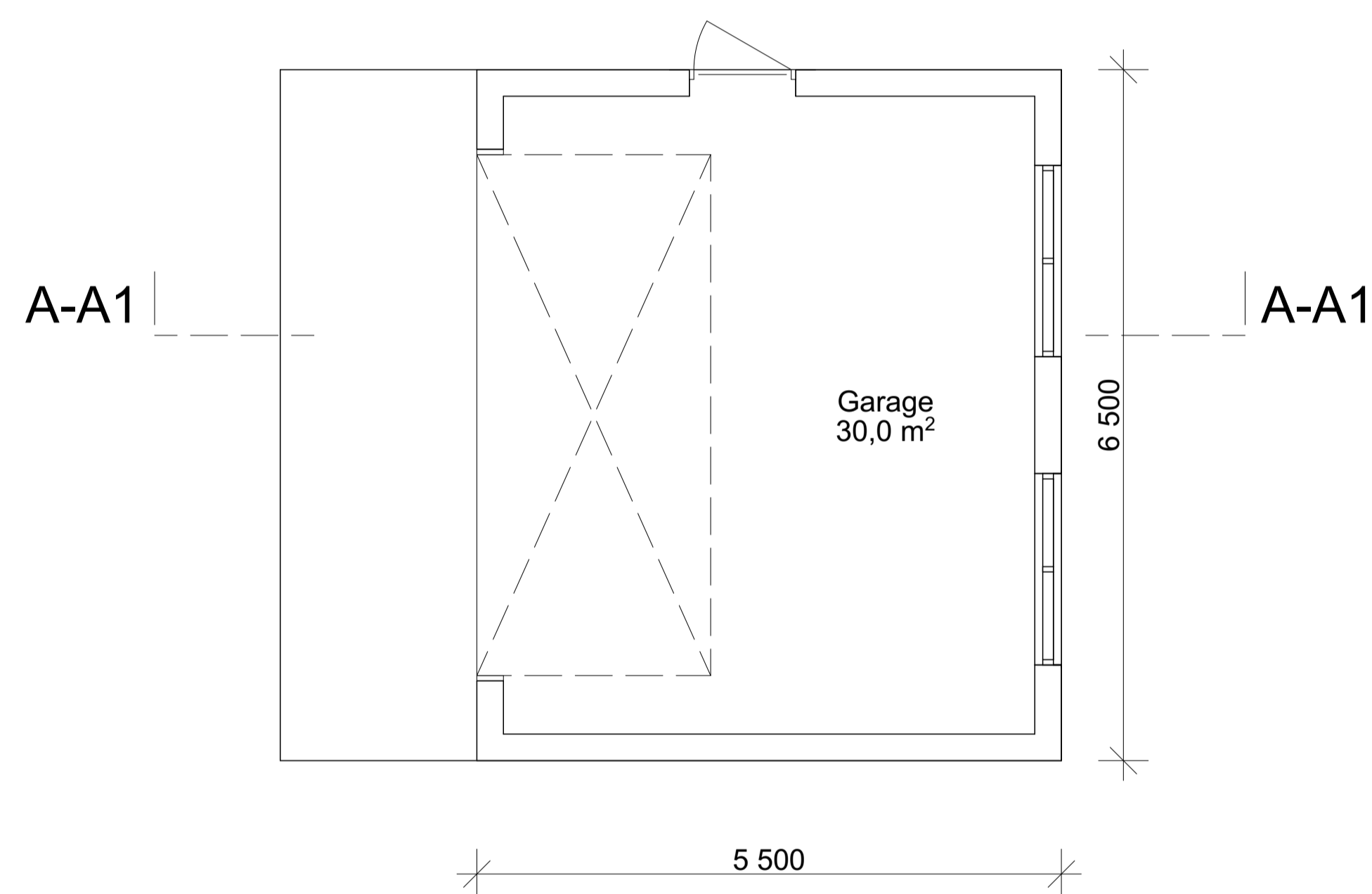
PLAN Byggnadsarea 35,7 m 2
