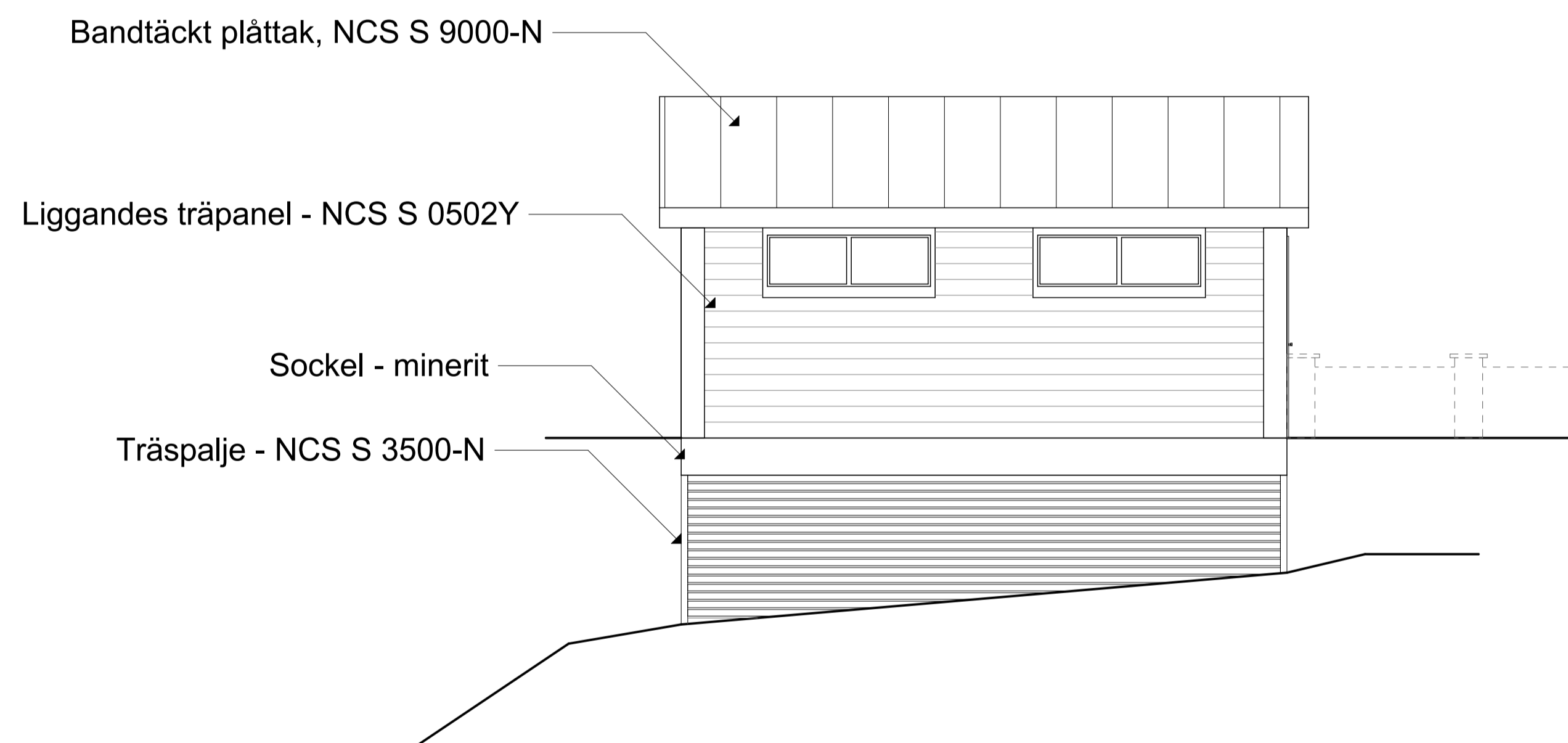
FASAD MOT NORR
