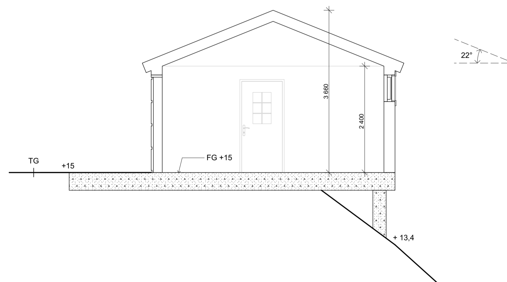
SEKTION A-A
