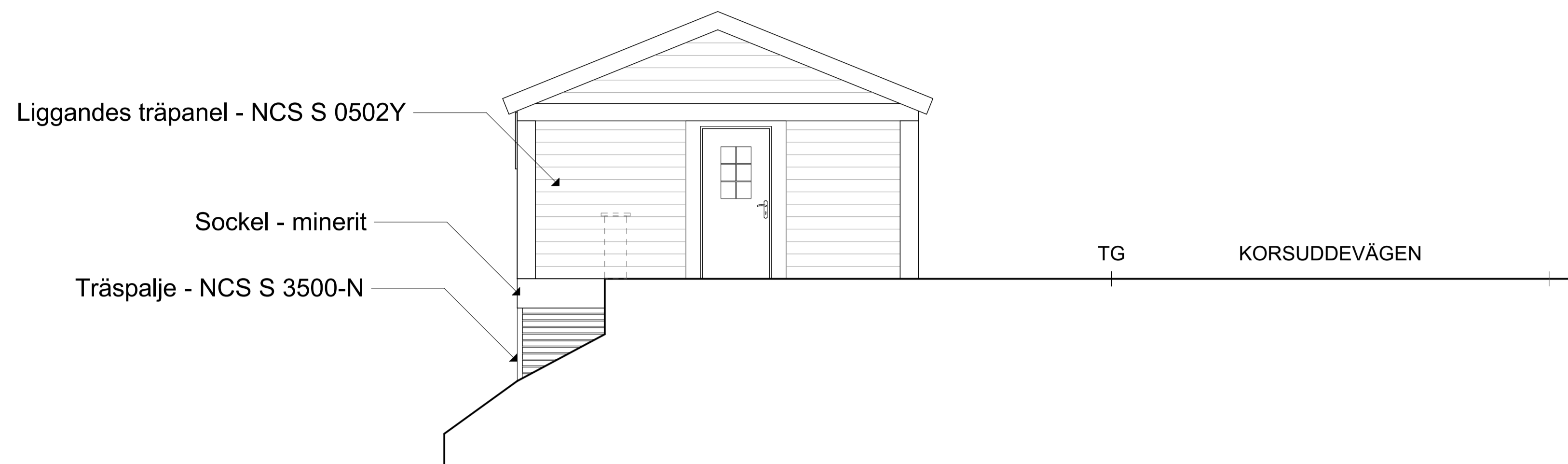
FASAD MOT VÄSTER
