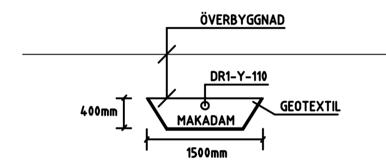
DETALJ MAKADAMBÄDD
