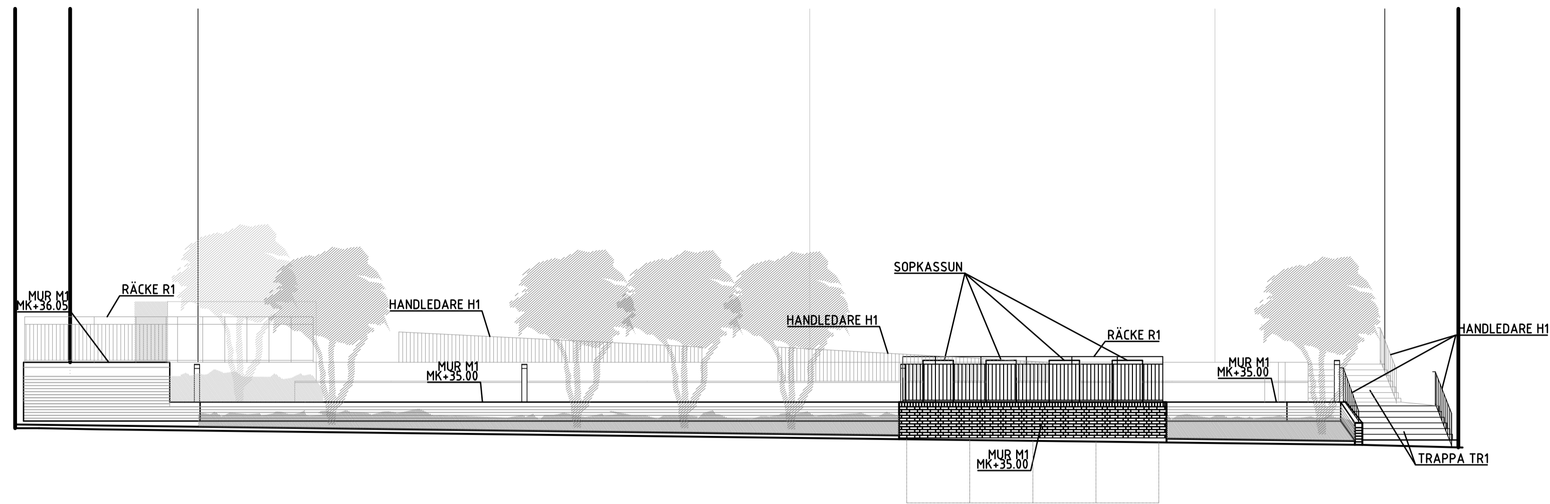
ELEVATION A-A
