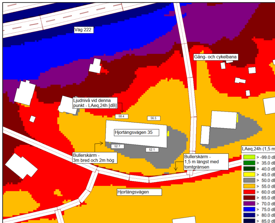
Figur 8. Bullerkarta över Hjortängsvägen 30 vid 1,5 m höjd. Ljudnivåskillnaden mellan skyddad och oskyddad sida är ca 5 dB. En 1,5 m hög bullerskärm längst med tomtrönsen mot Hjortängsvägen är inlagd i modellen.
