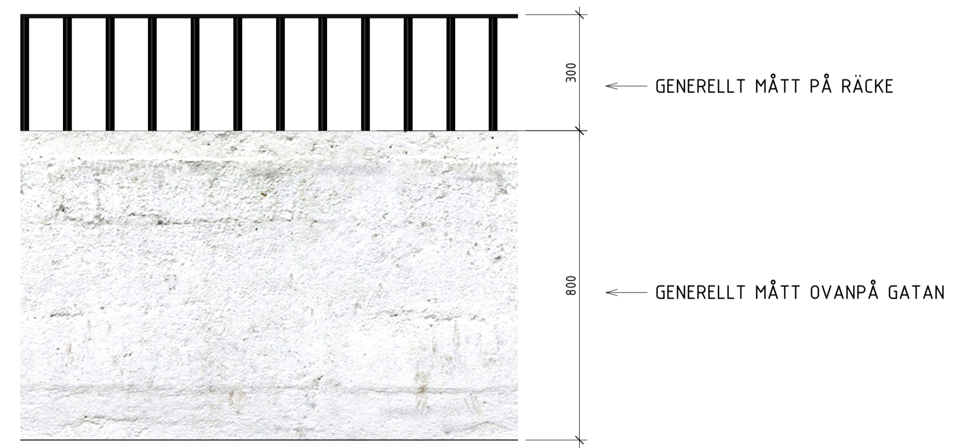
DETALJ A-A SKALA 1:10 (A1)
