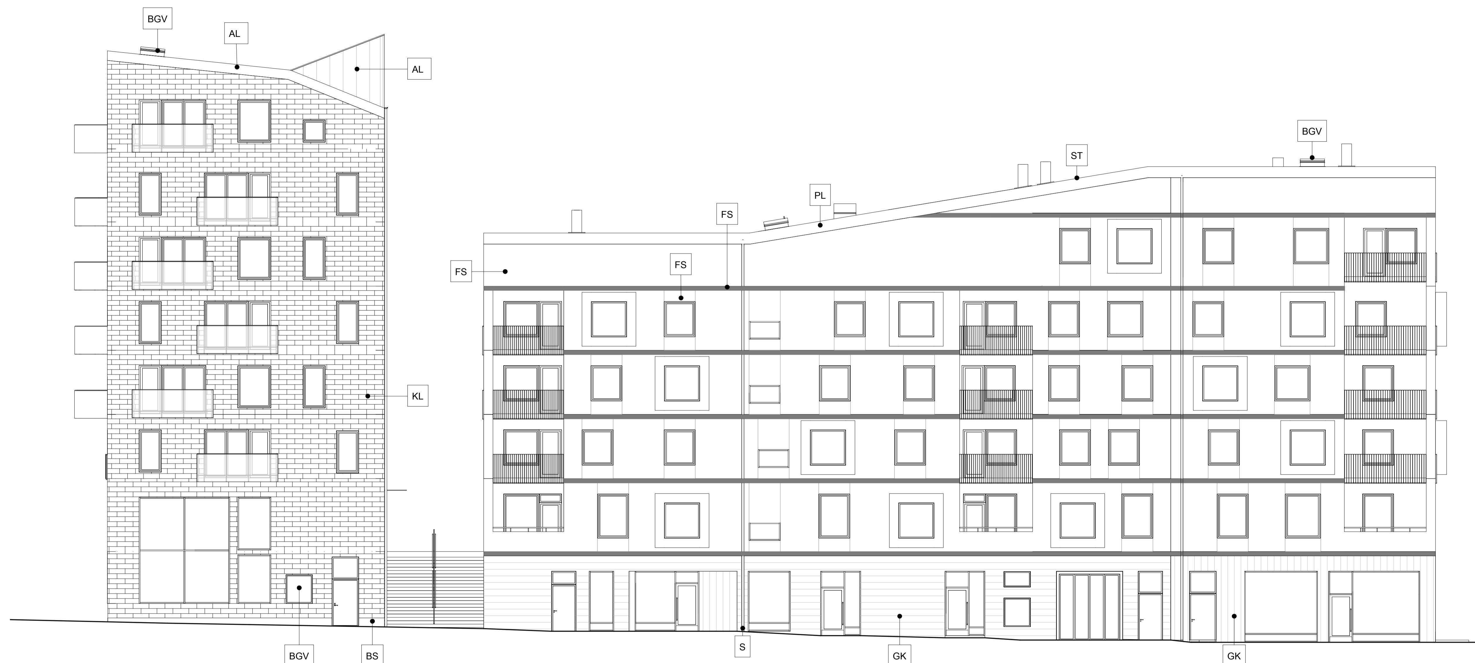
Fasad mot sydöst SKALA 1 : 100
