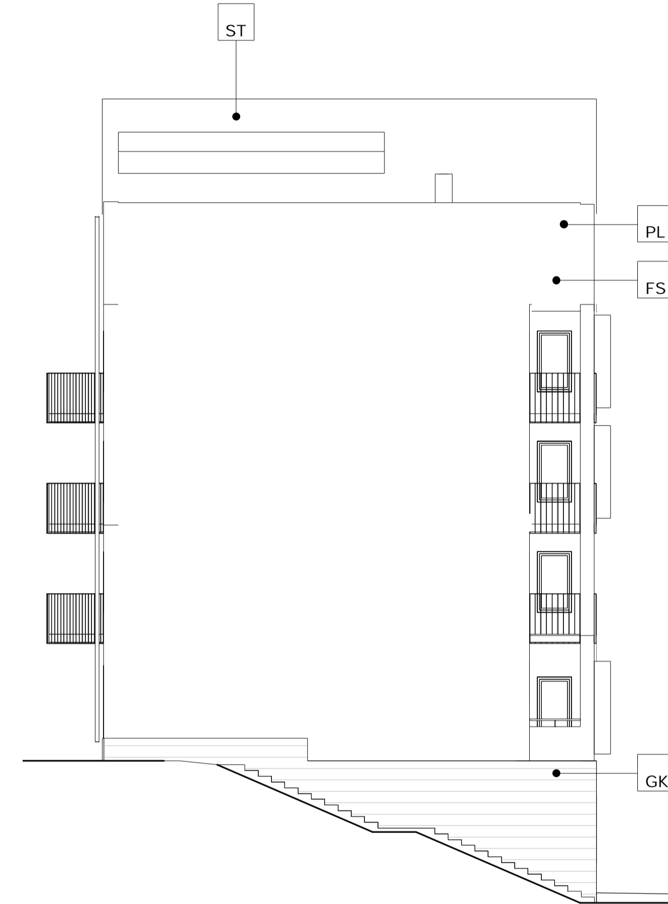
Gårdsfasad mot Sydväst 2 SKALA 1 : 100
