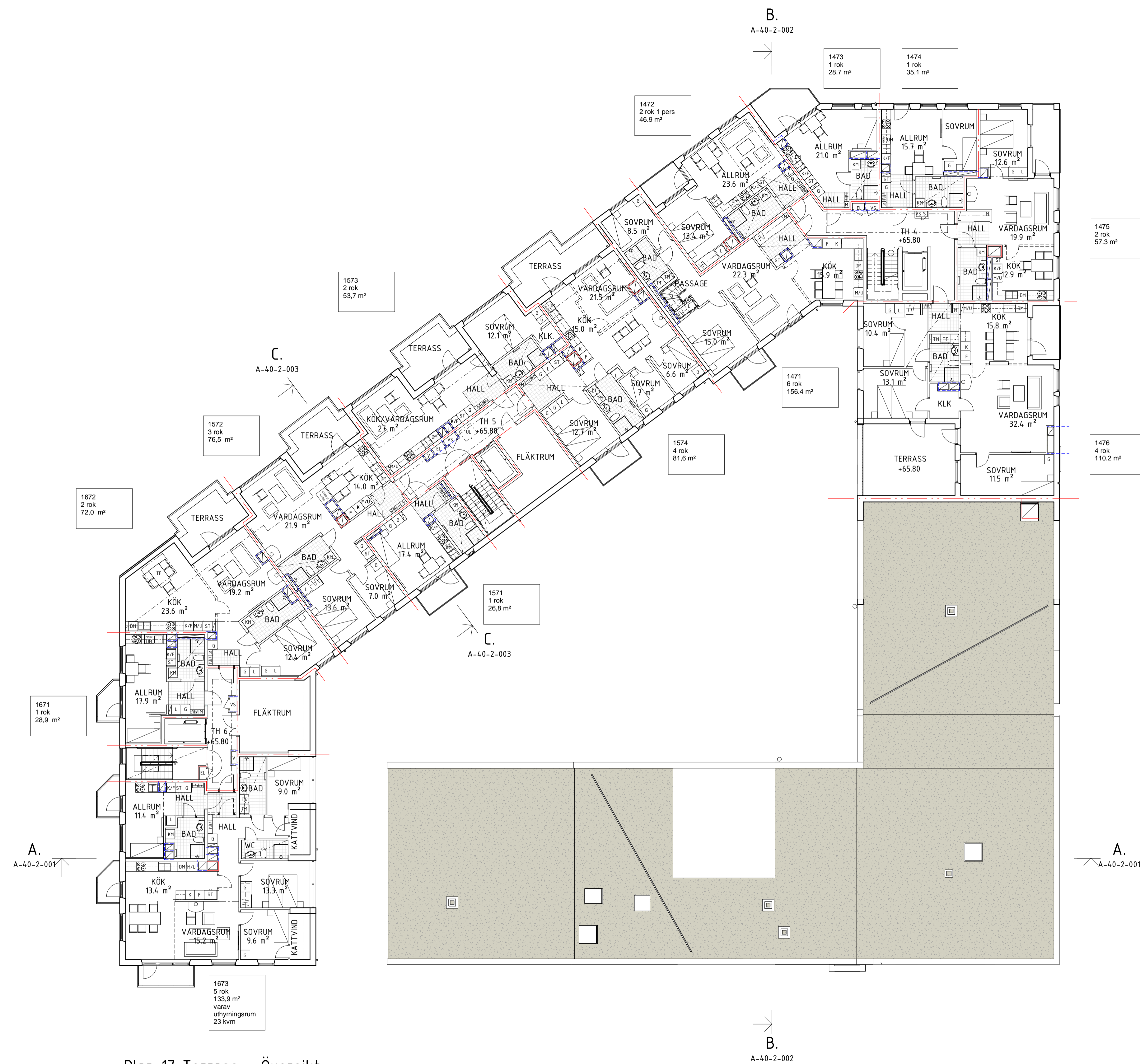
Plan 17 Terrass - Översikt
