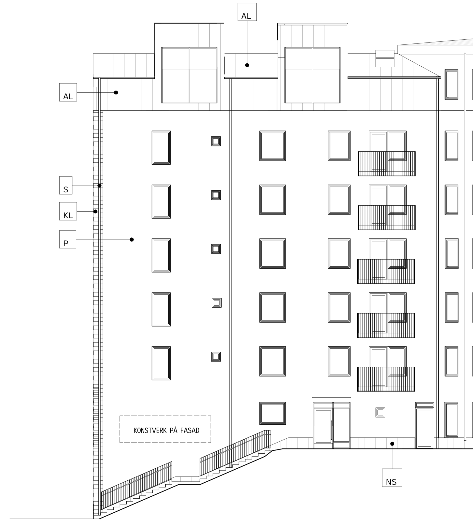
Gårdfasad mot Nordöst SKALA 1 : 100
