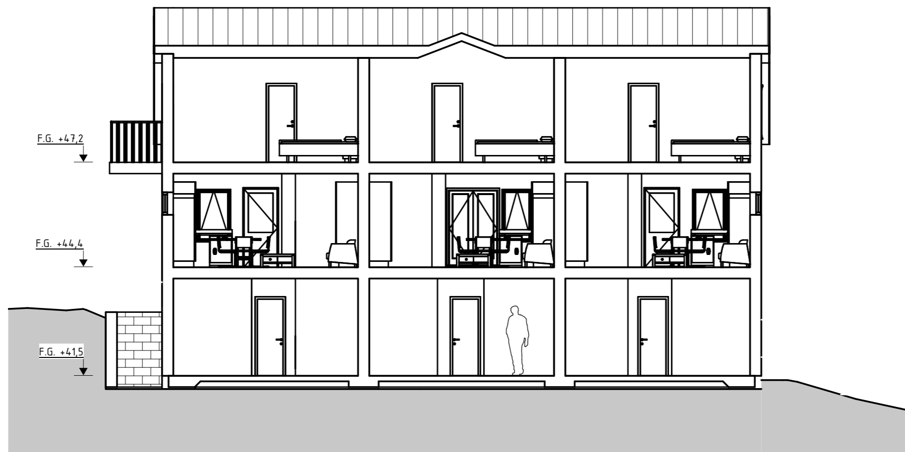
SEKTION B-B
