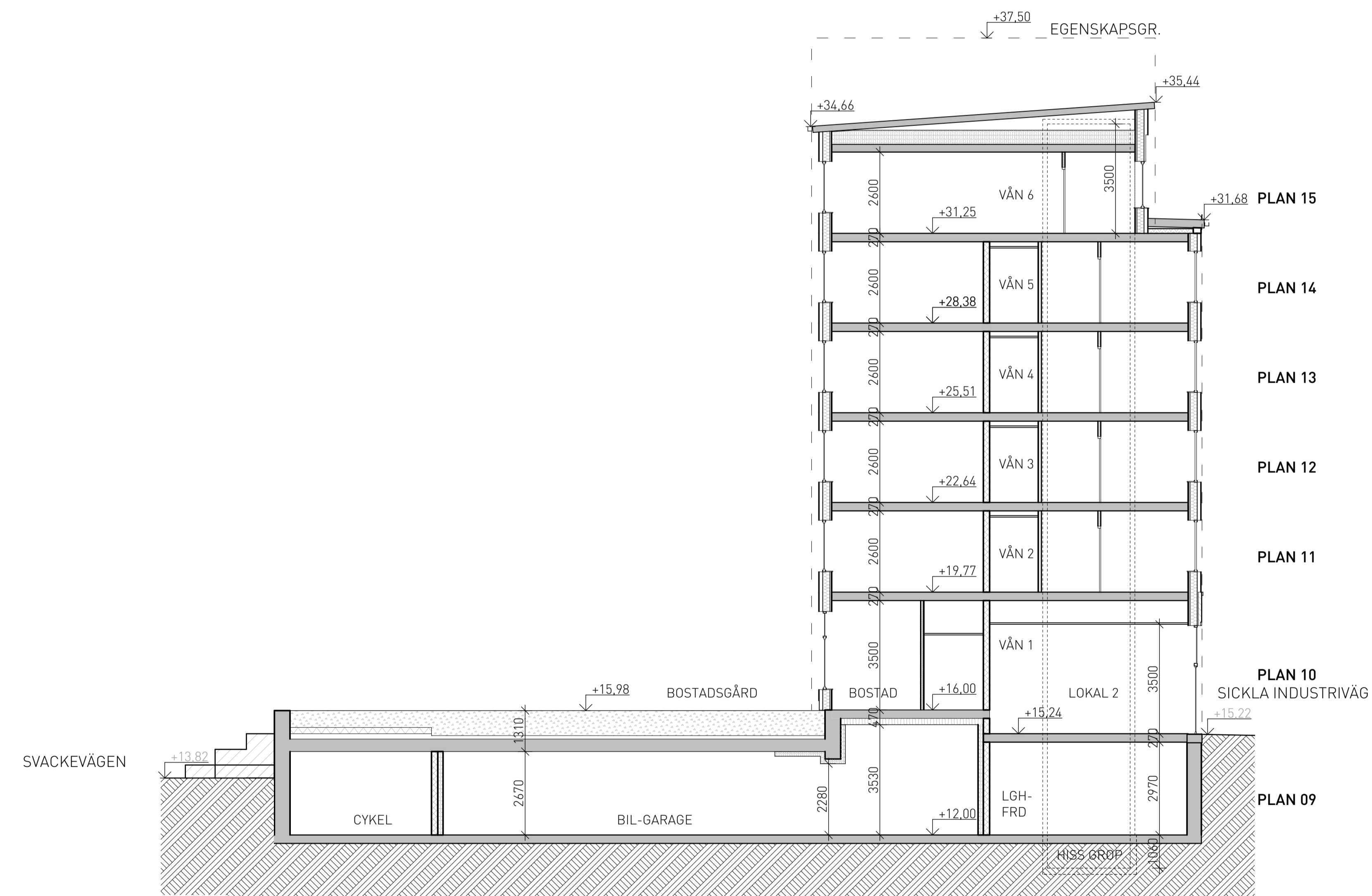
TVÄRSEKTION B-B
