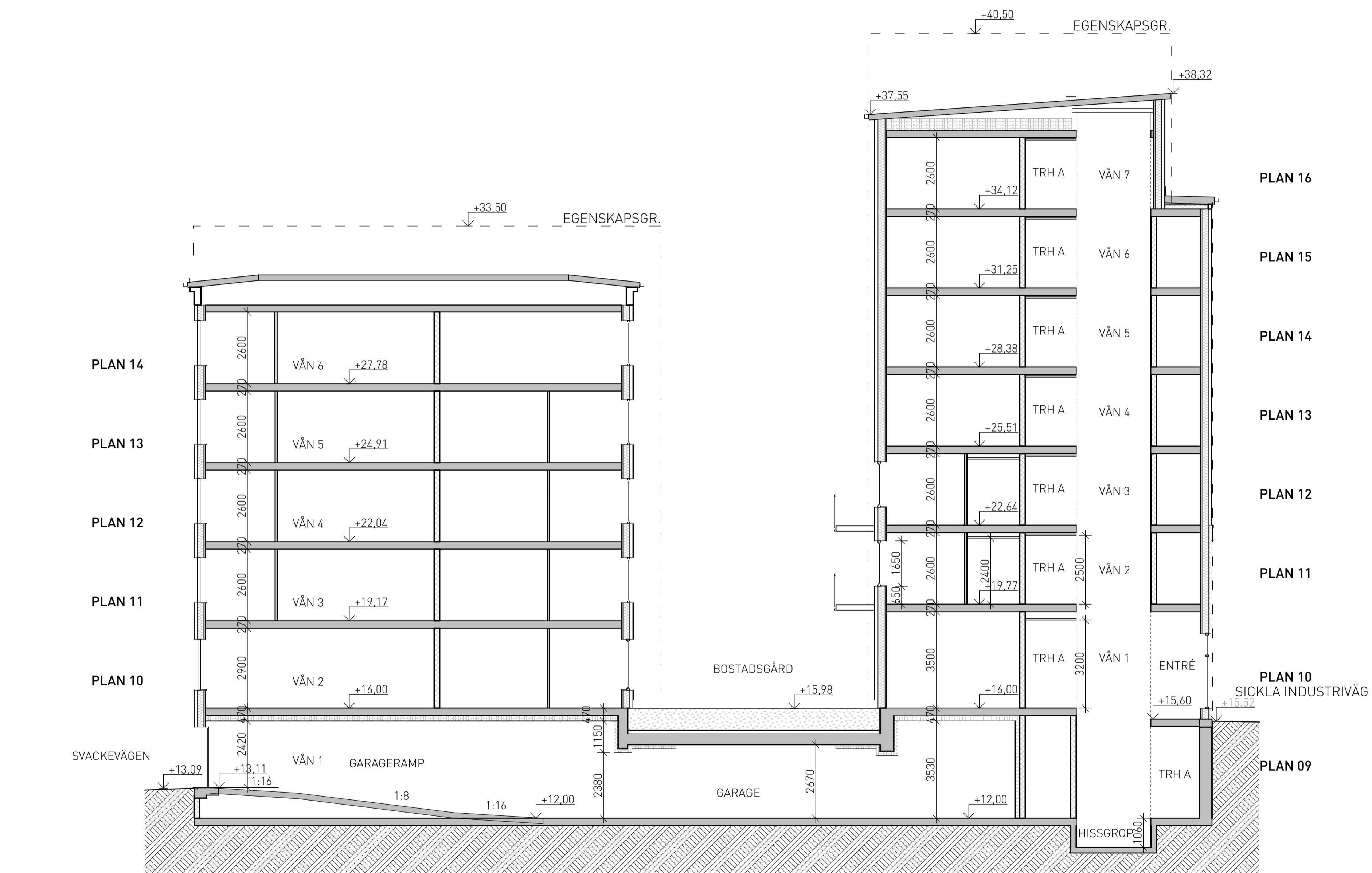
TVÄRSEKTION D-D
