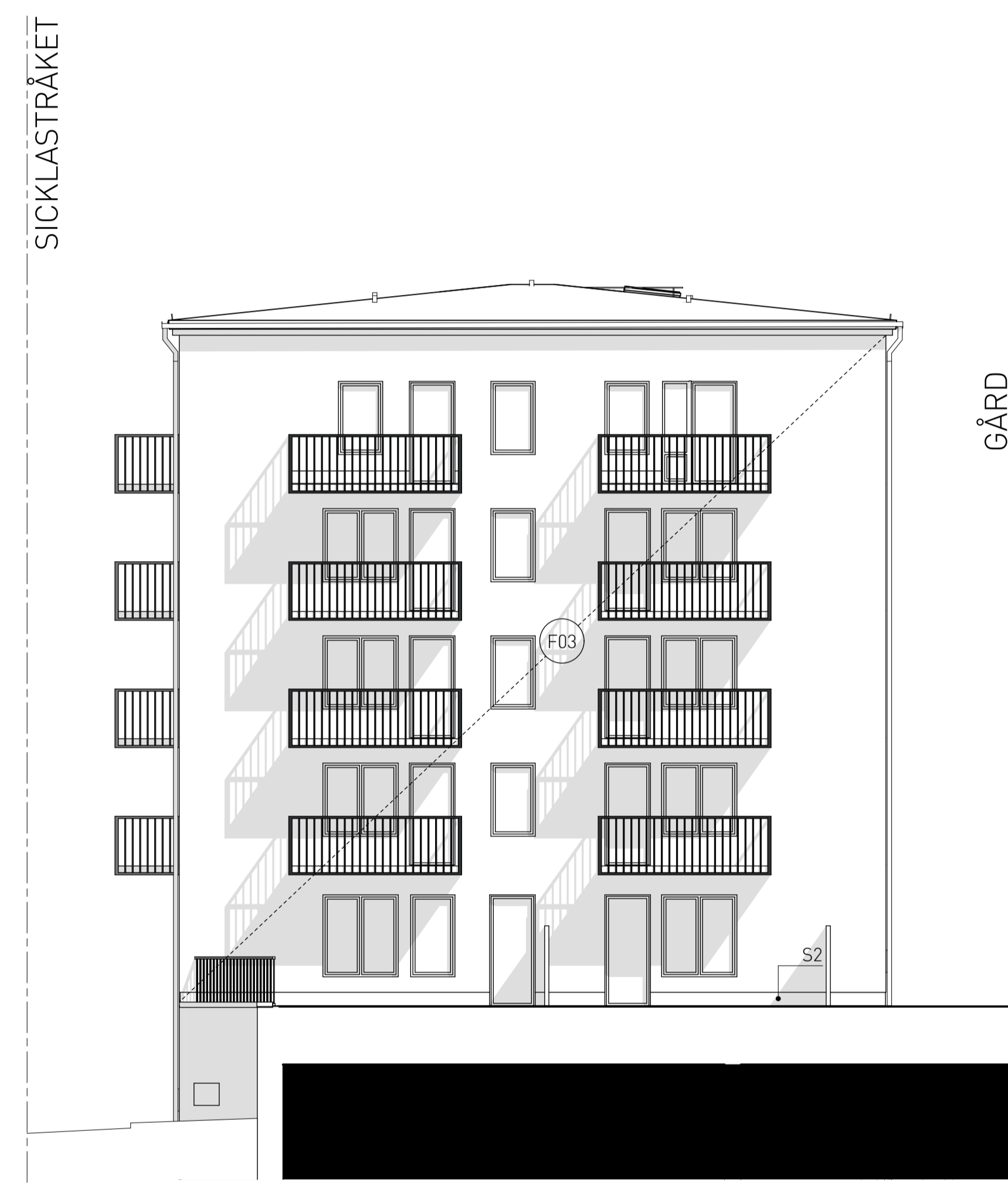
FASAD FÄRG/SV GÅRDSFASAD HUS C (SÖDER) 1:100
