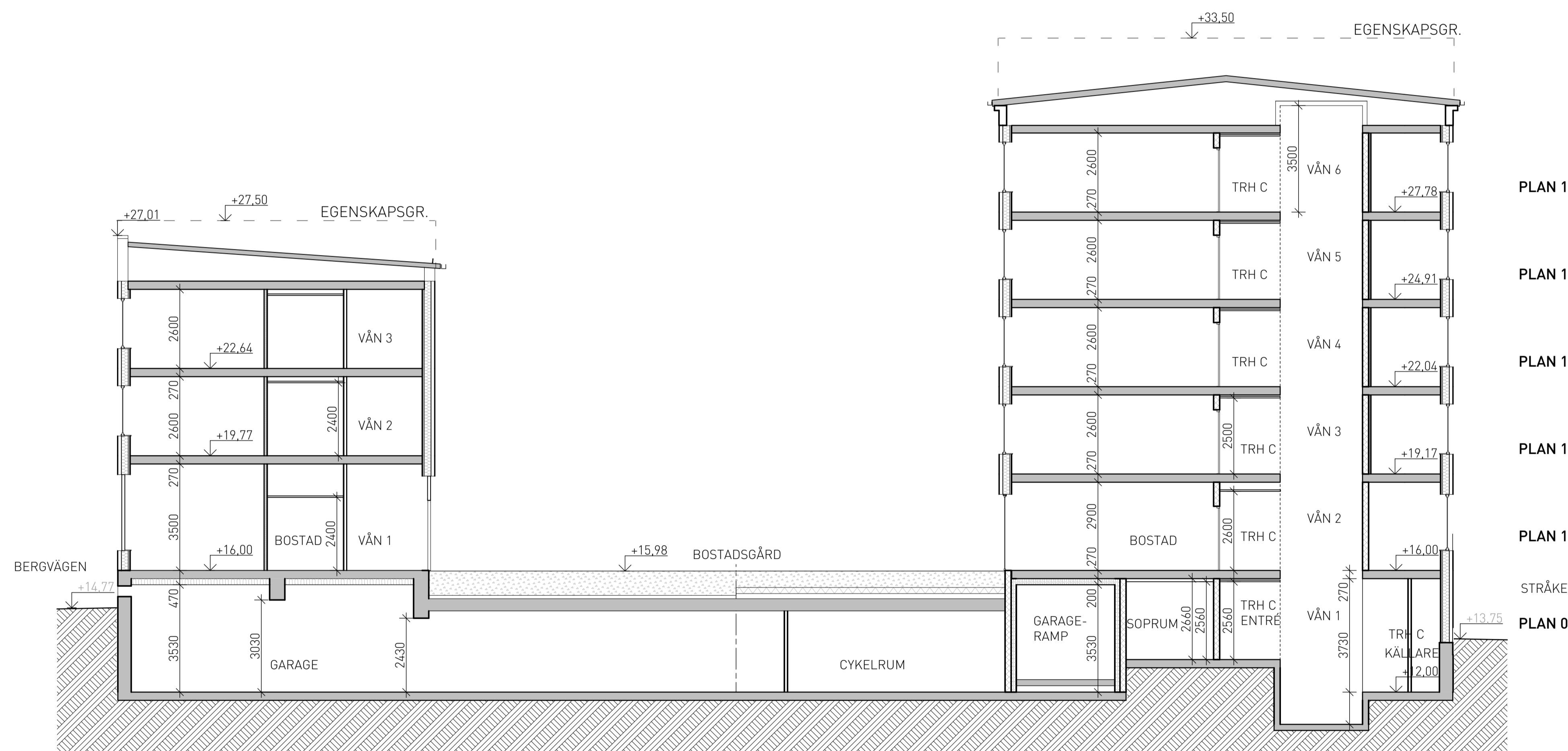
LÅNGDSEKTION 2-2
