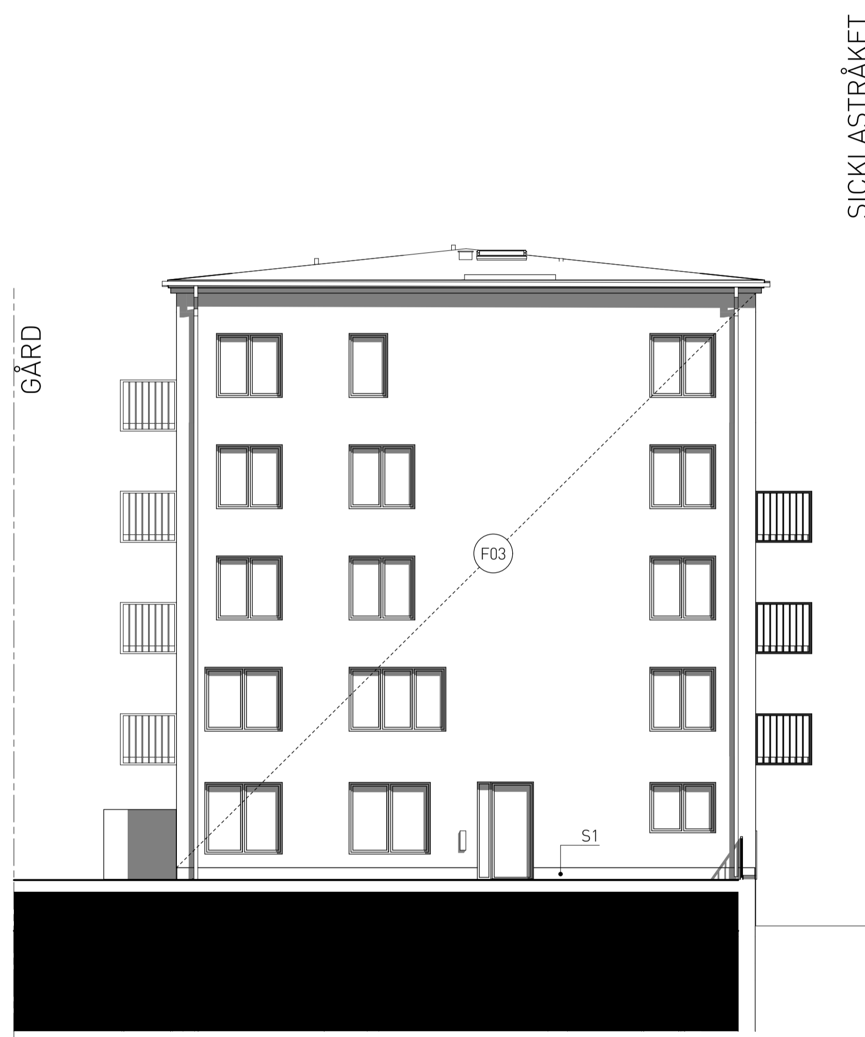
FASAD FÄRG/SV GÅRDSFASAD HUS C (ÖSTER) 1:100
