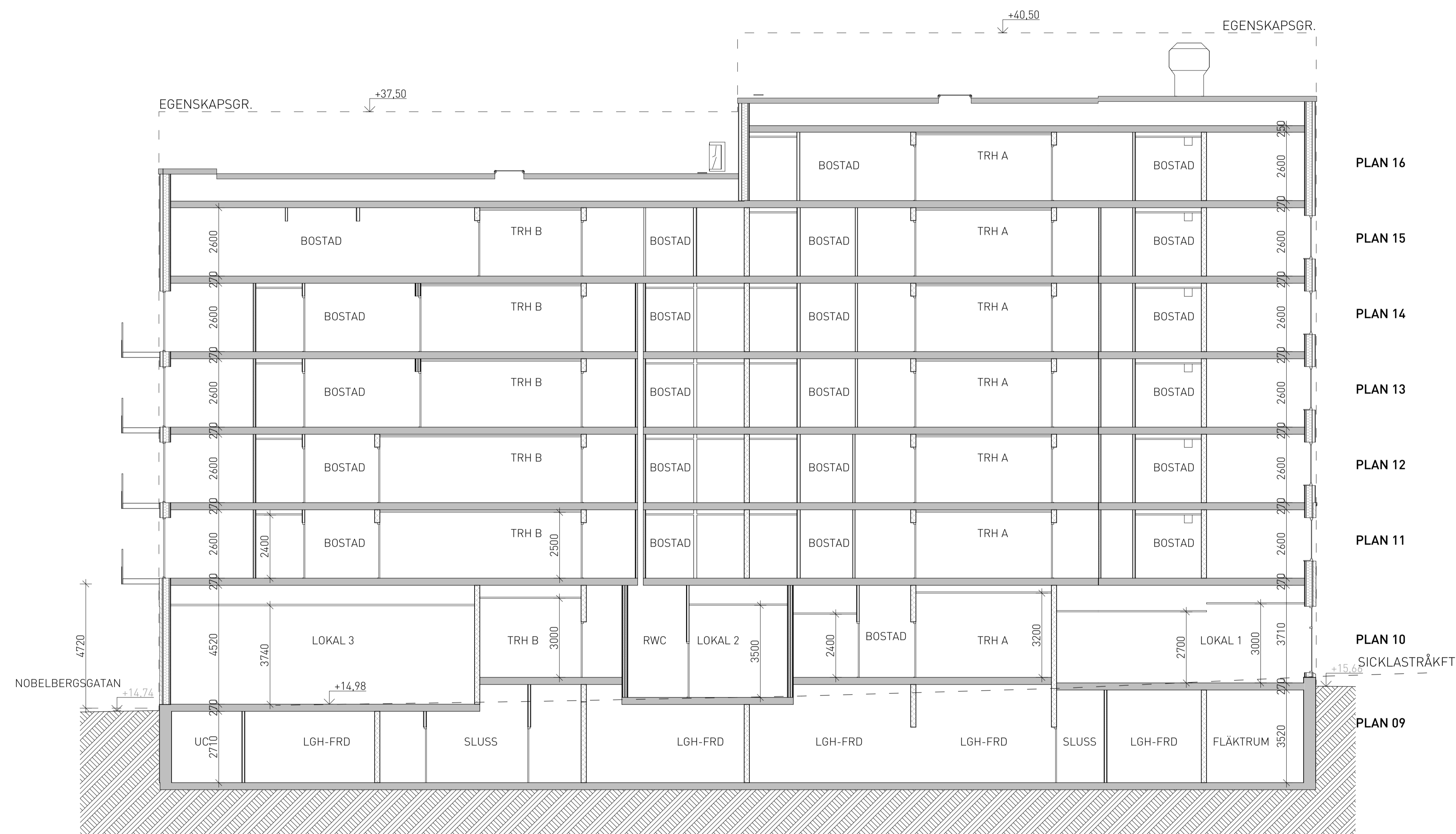
LÄNGDSEKTION 1-1
