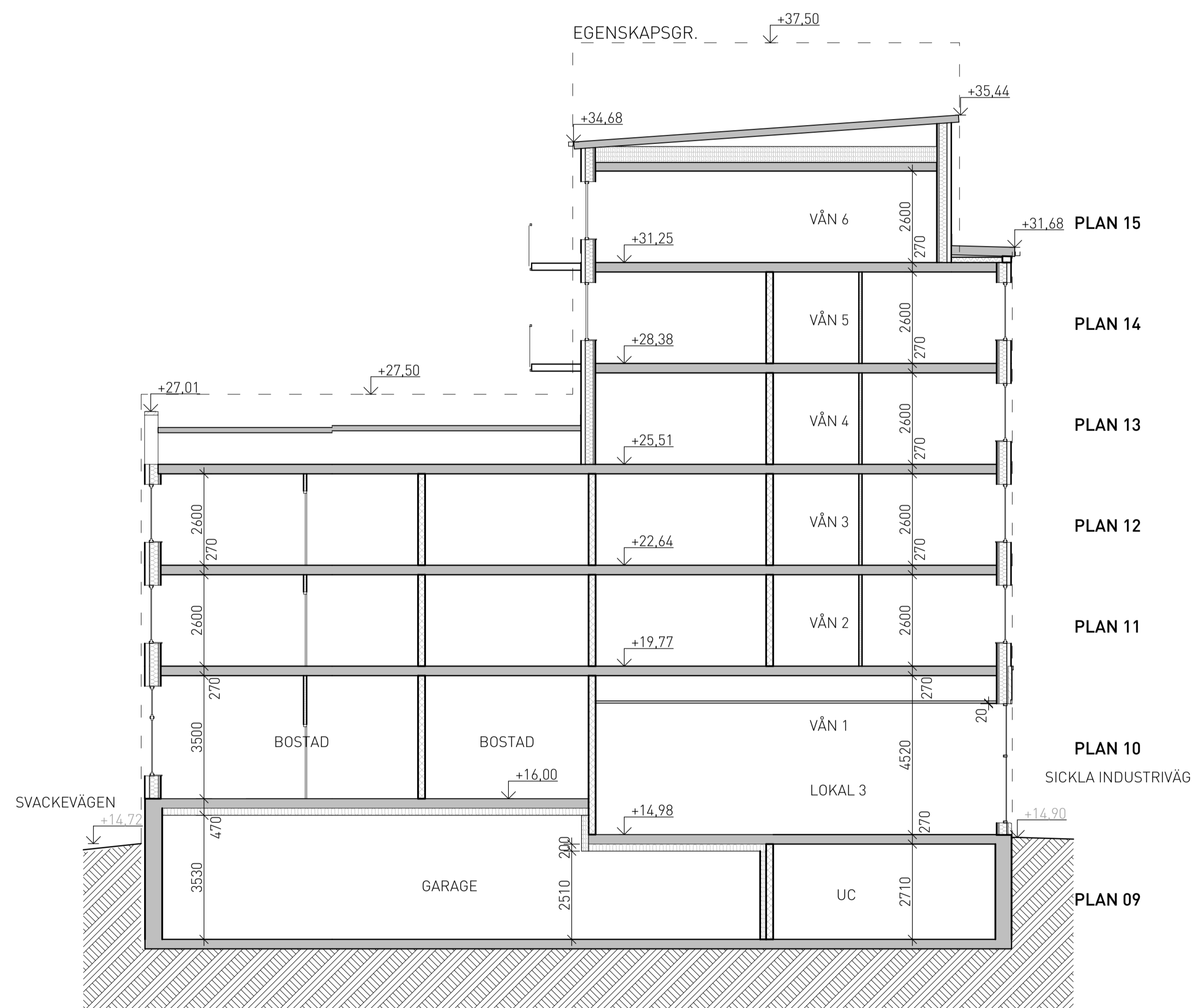
TVÄRSEKTION A-A
