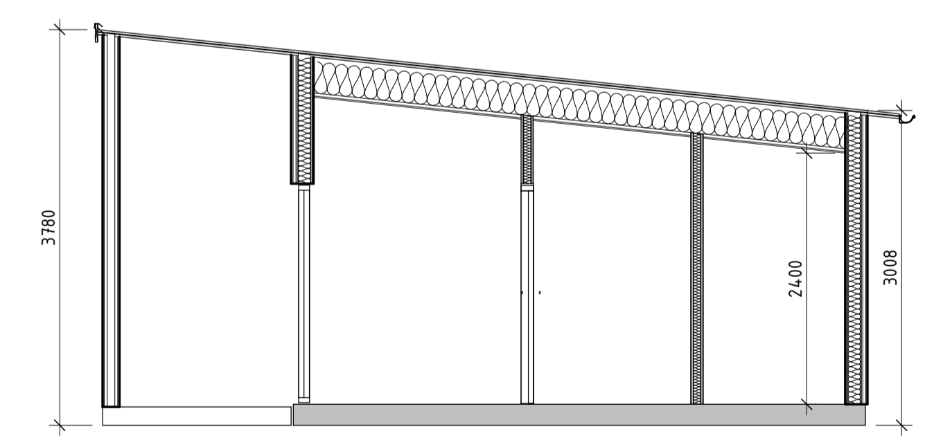
SEKTION A-A
