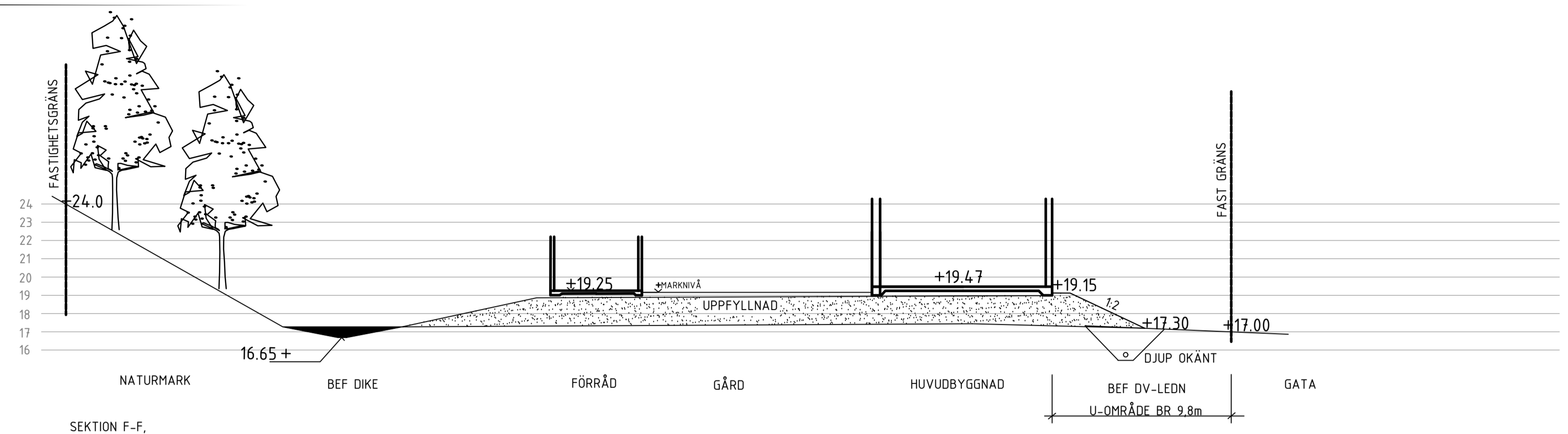
SEKTION F-F, SKALA 1:200 (A1)
