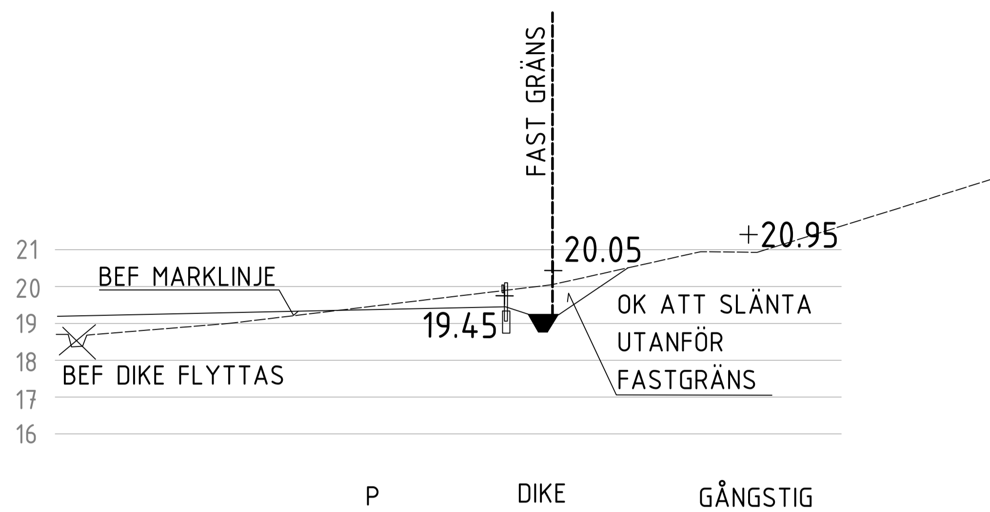
SEKTION E-E, SKALA 1:100 (A1)
