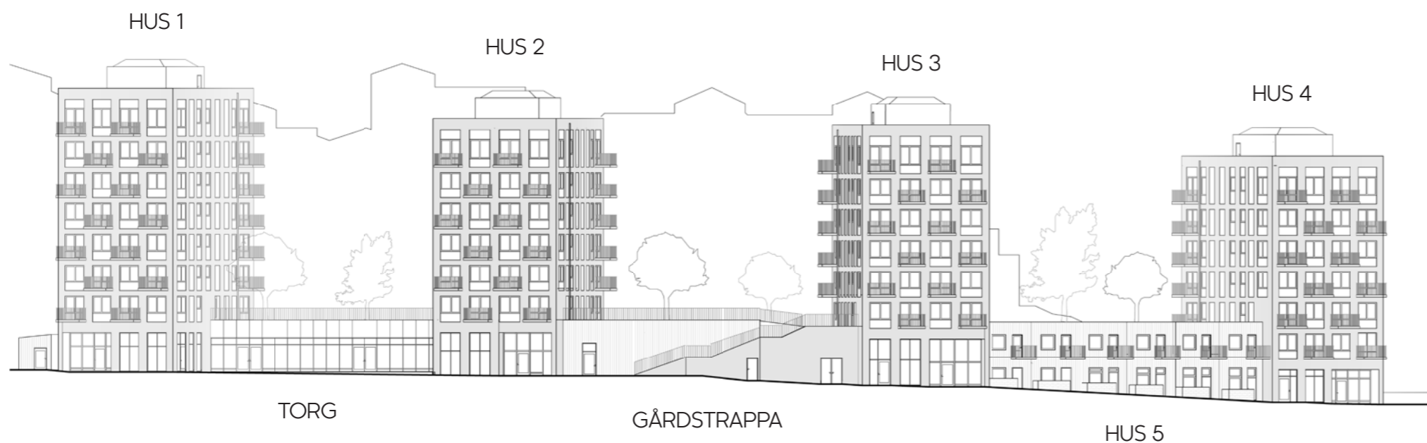
Princip - fasadens gridsystem med ramverk av tegel, intryck med puts och plåtavtäckningar vid fönster.
