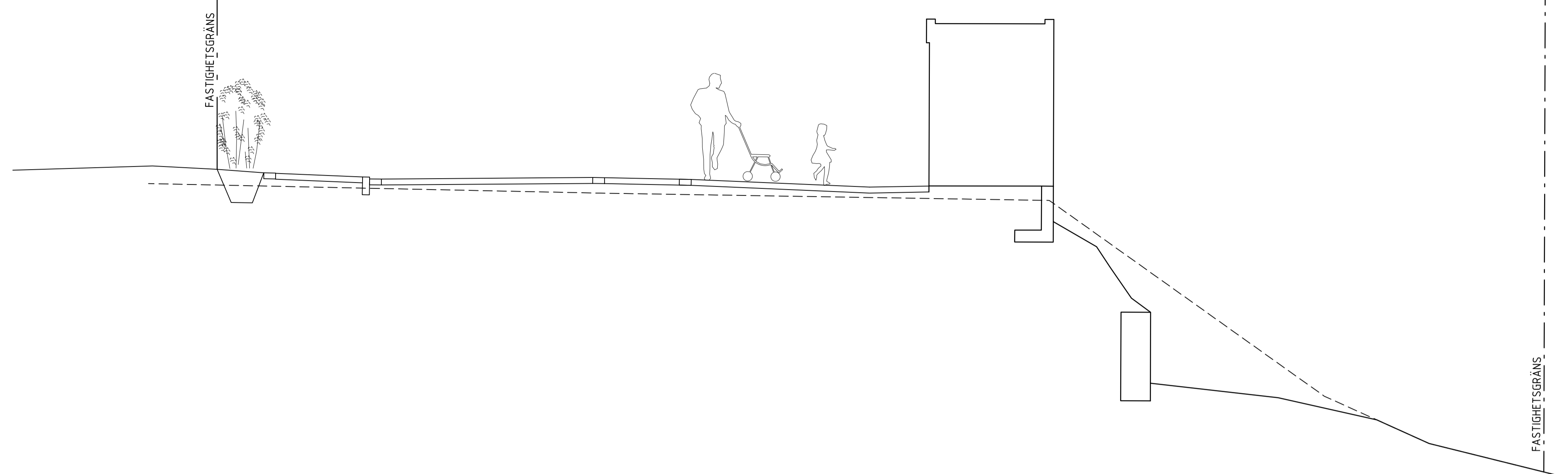
SEKTION Q-q 1:50(A1) / 1:100(A3)
