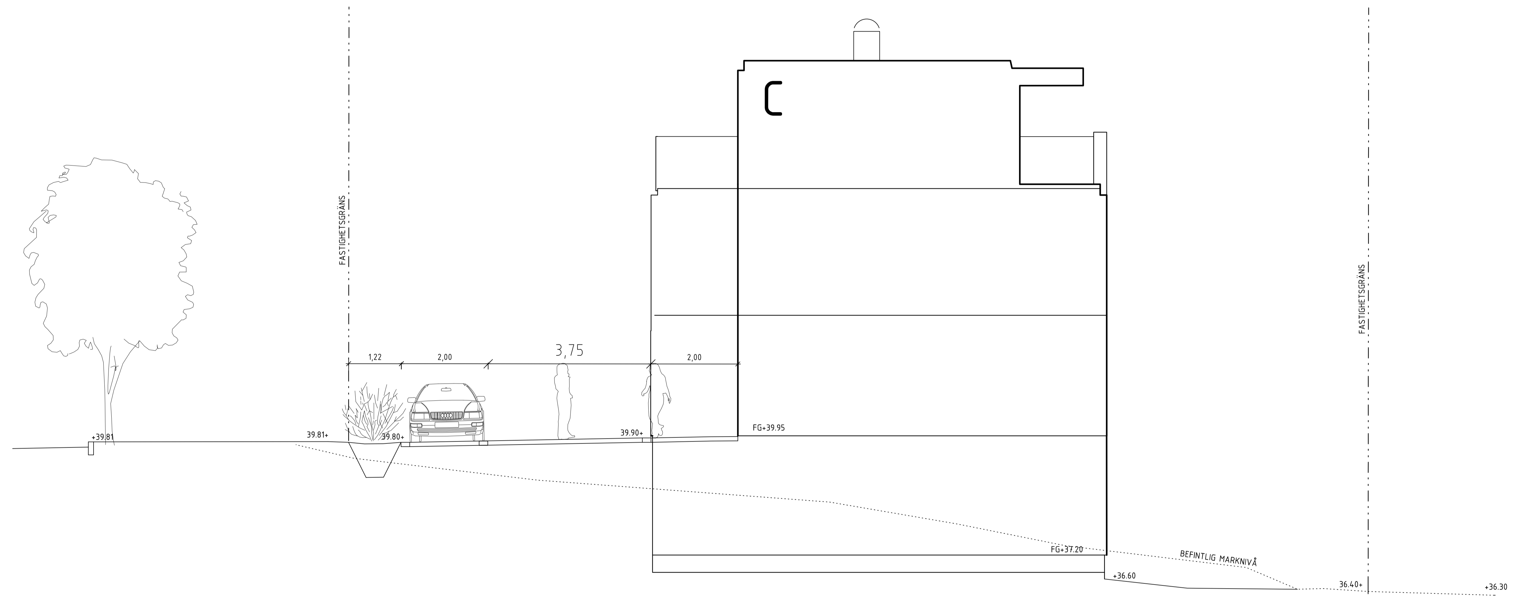
SEKTION A-a 1:50(A1) / 1:100(A3)
