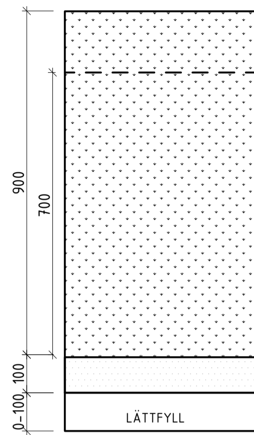
PL6 PLANTERINGSYTA PÅ BJÄLKLAG FÖR TRÄD, BUSKAR OCH PERENNER
