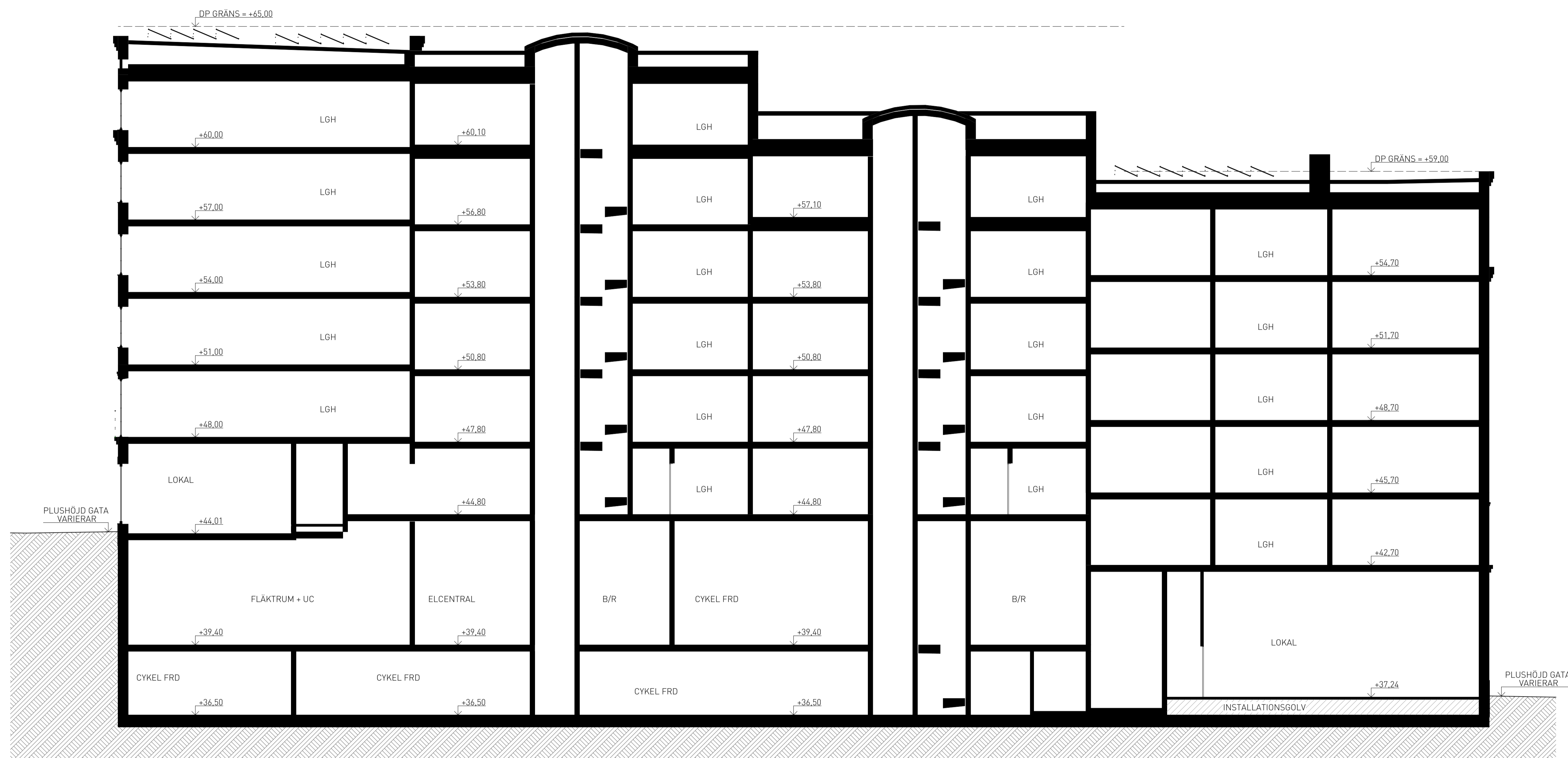
Sektion E-E 1:100
