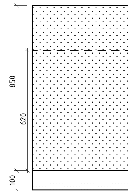
PL5 PLANTERINGSYTA PÅ BJÄLKLAG PERENNER OCH BUSKAR
