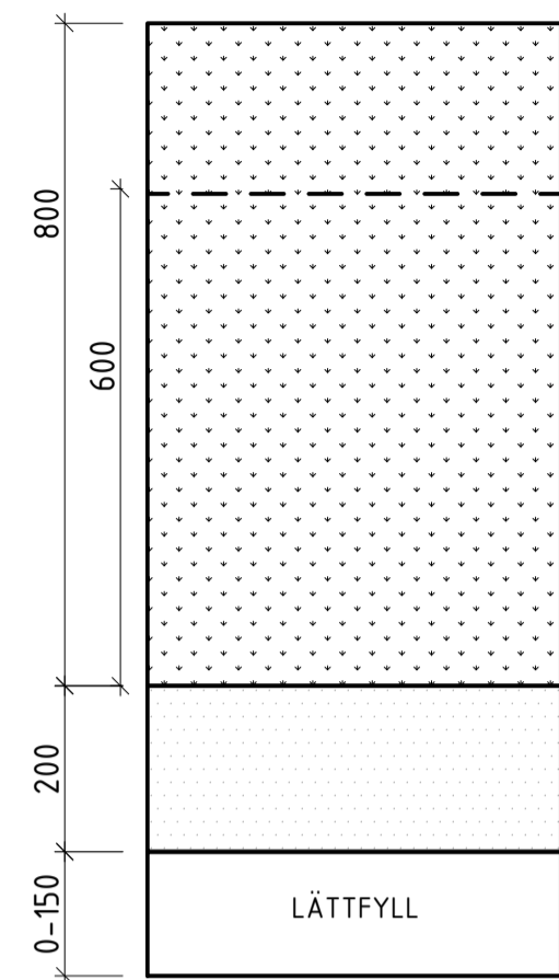
PL4 REGNBÄDD PÅ BJÄLKLAG FÖR TRÄD, BUSKAR OCH PERENNER
