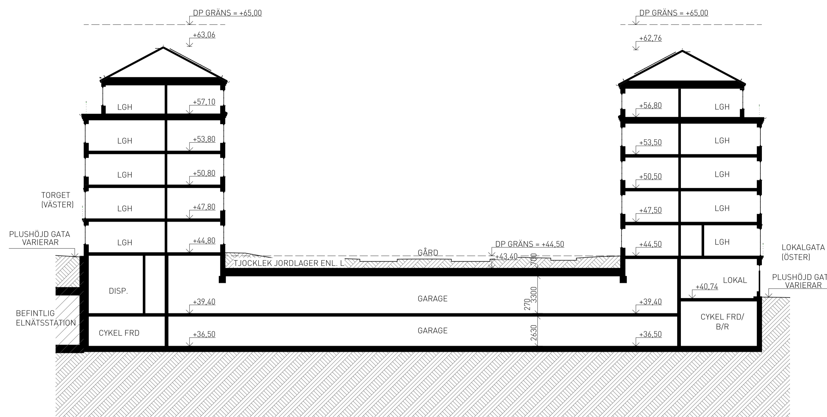
Sektion A-A 1:200
