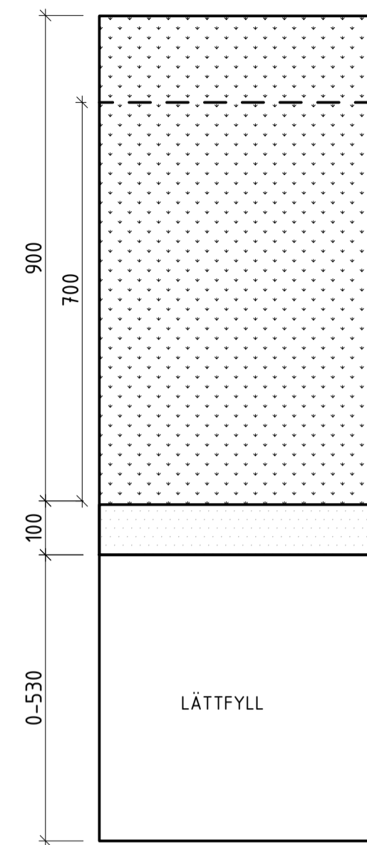
PL1-3 PLANTERINGSYTA PÅ BJÄLKLAG FÖR TRÄD, BUSKAR OCH PERENNER
