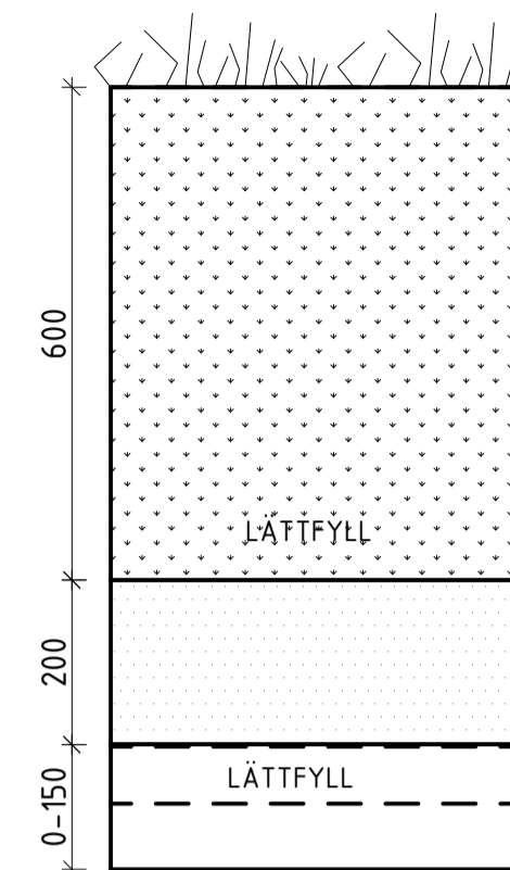
GR1 GRÄSYTA PÅ BJÄLKLAG
