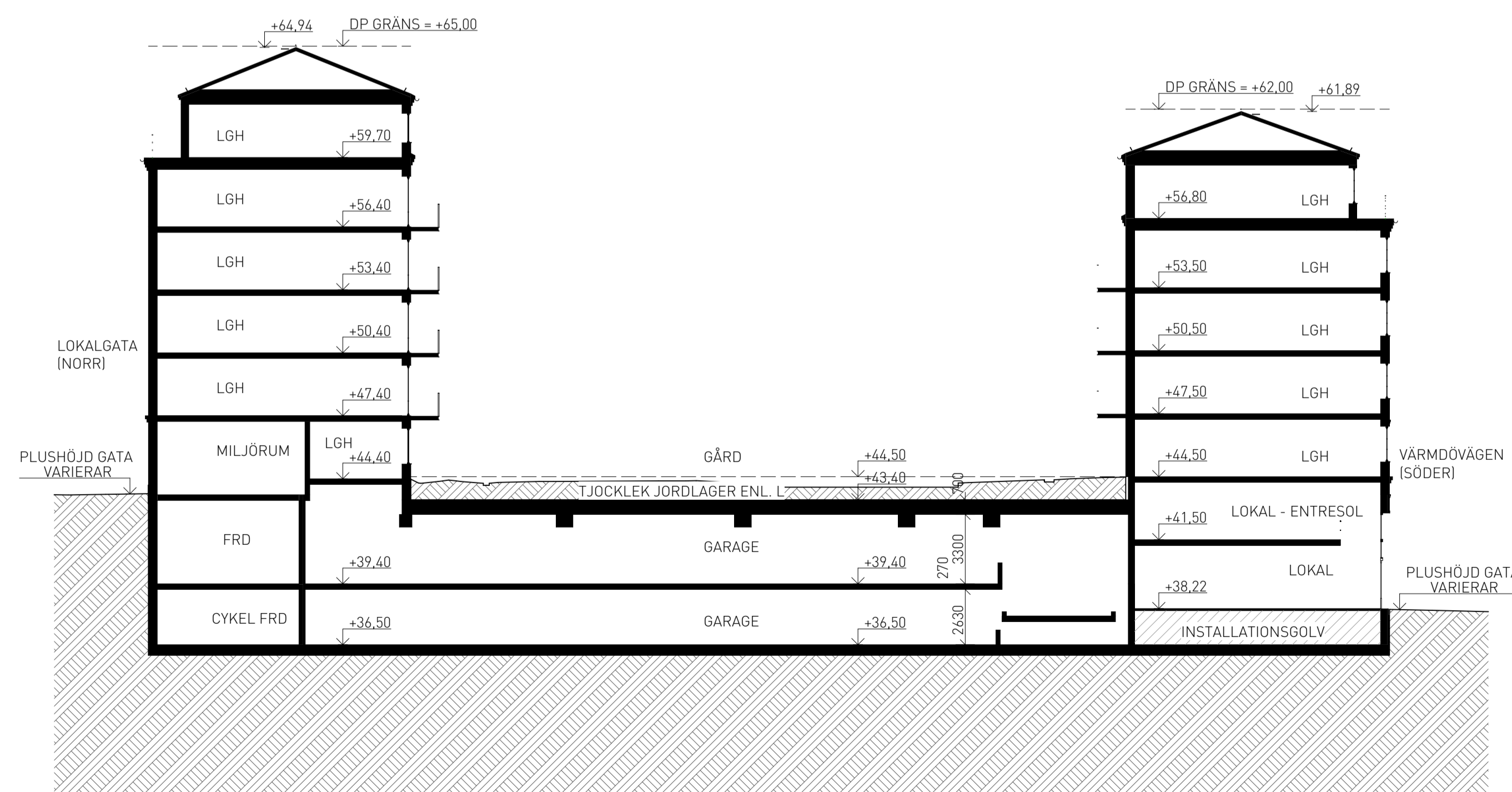
Sektion B-B 1:200
