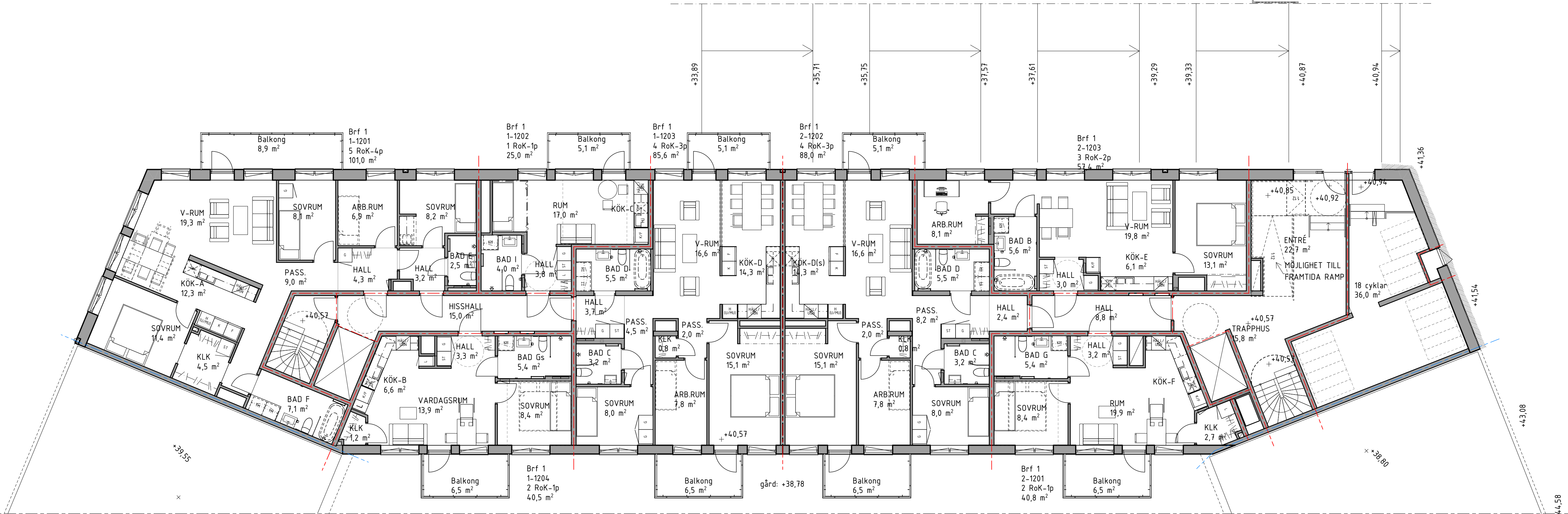
Plan 12 1:100
