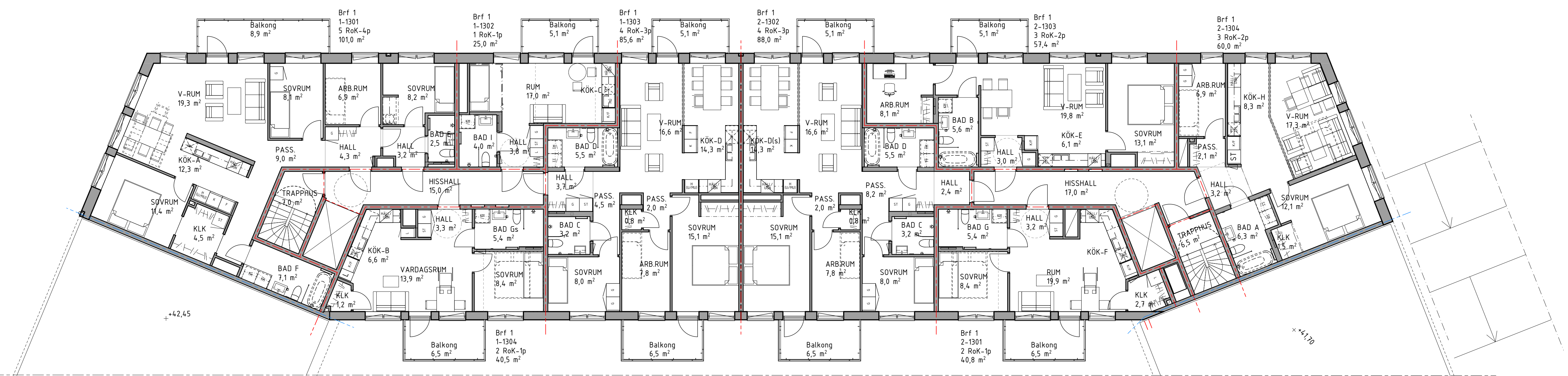
Plan 13 1:100
