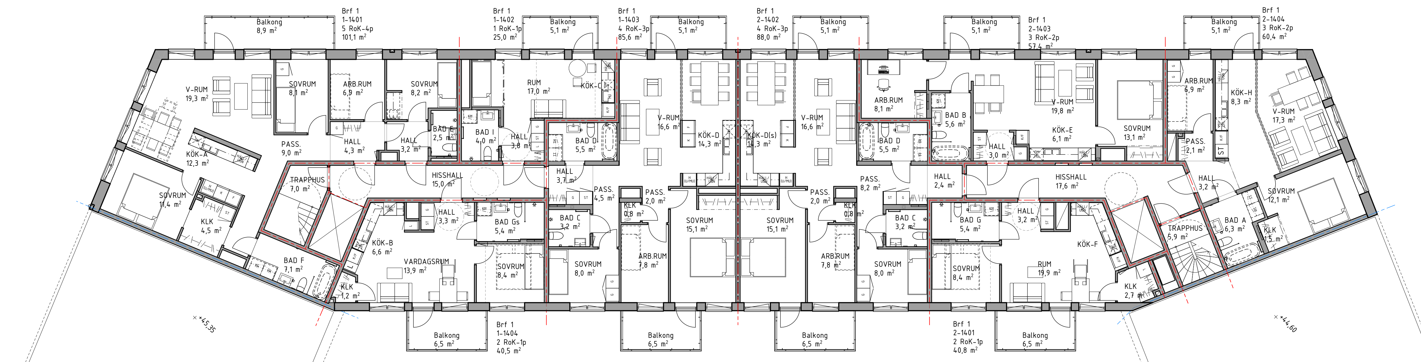
Plan 14 1:100
