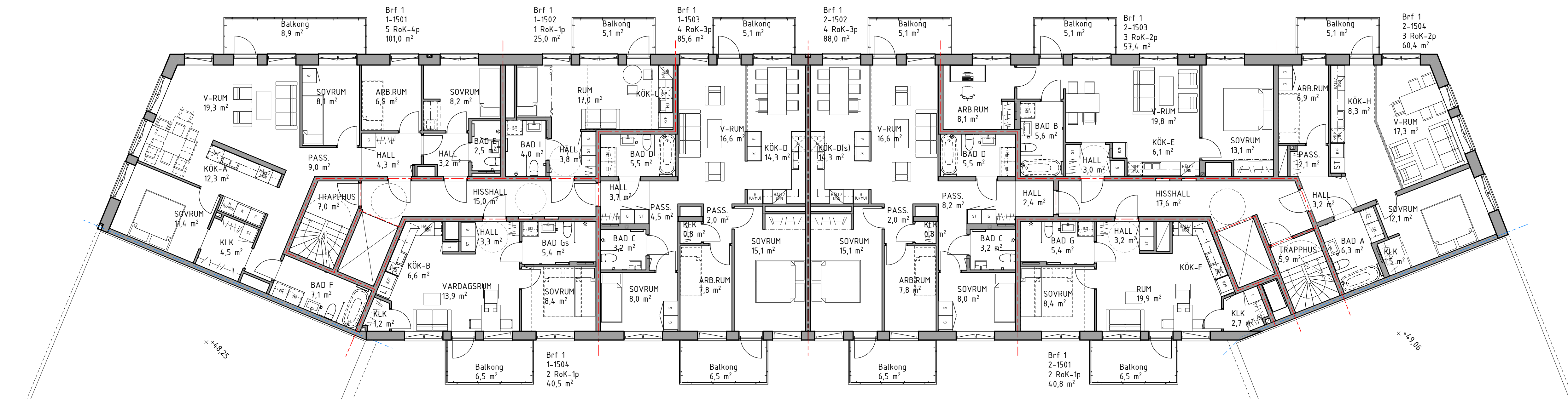
Plan 15 1:100
