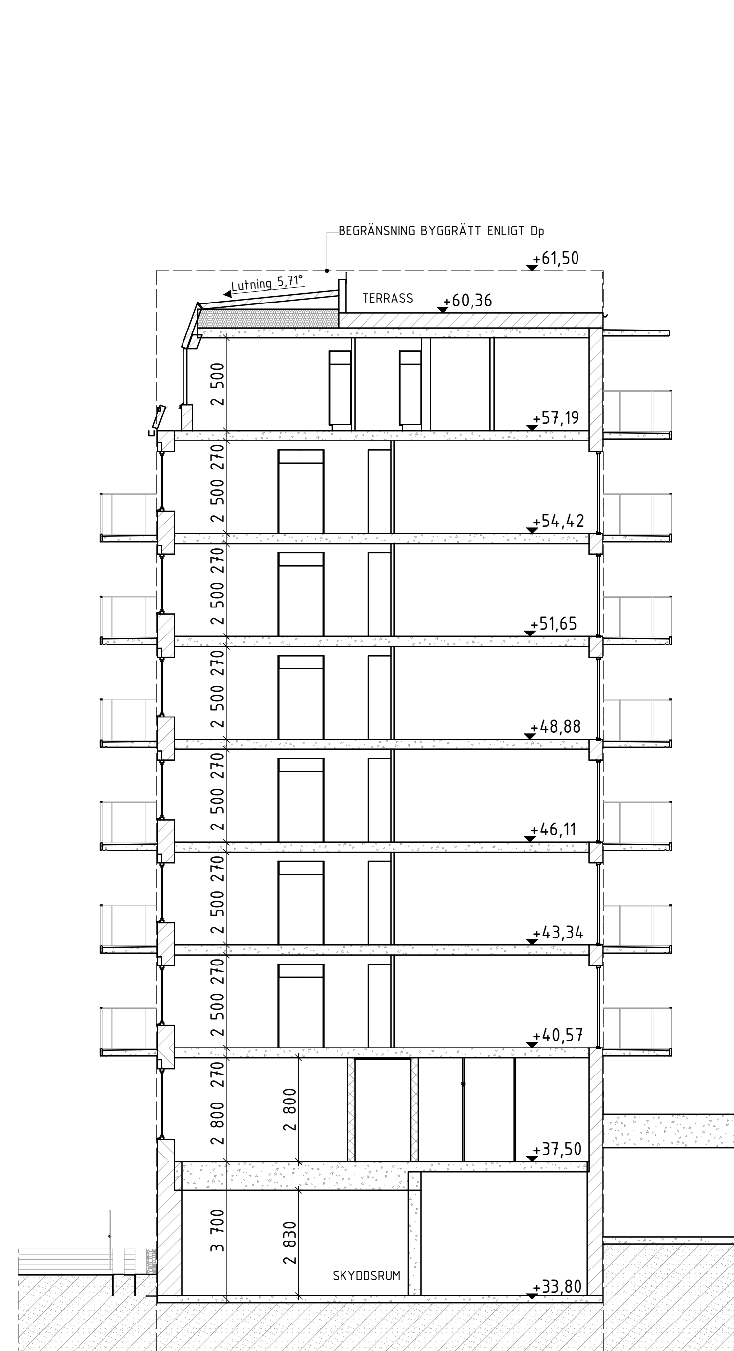
Tvärsektion 2 1:100
