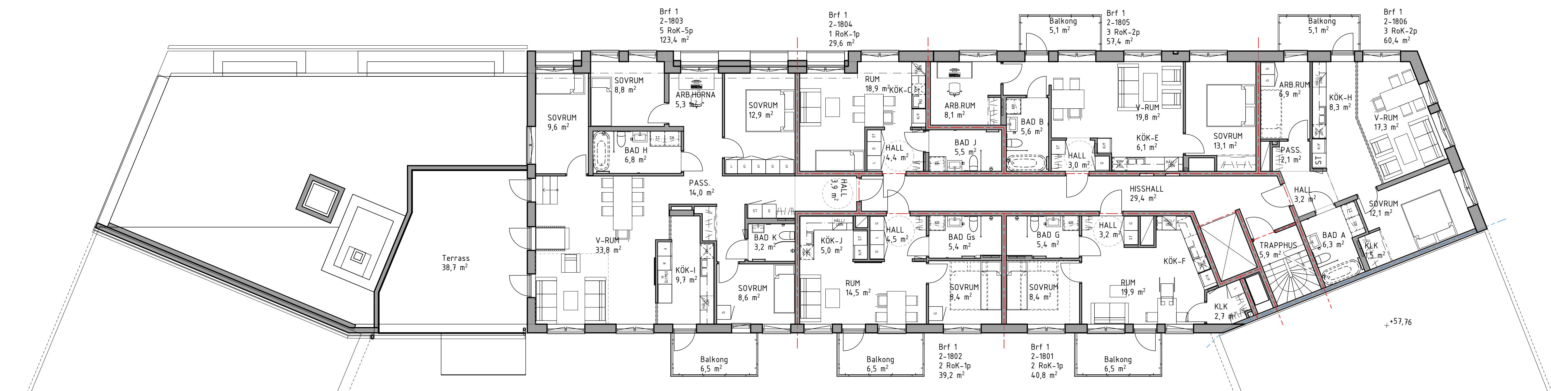
Plan 18 1:100
