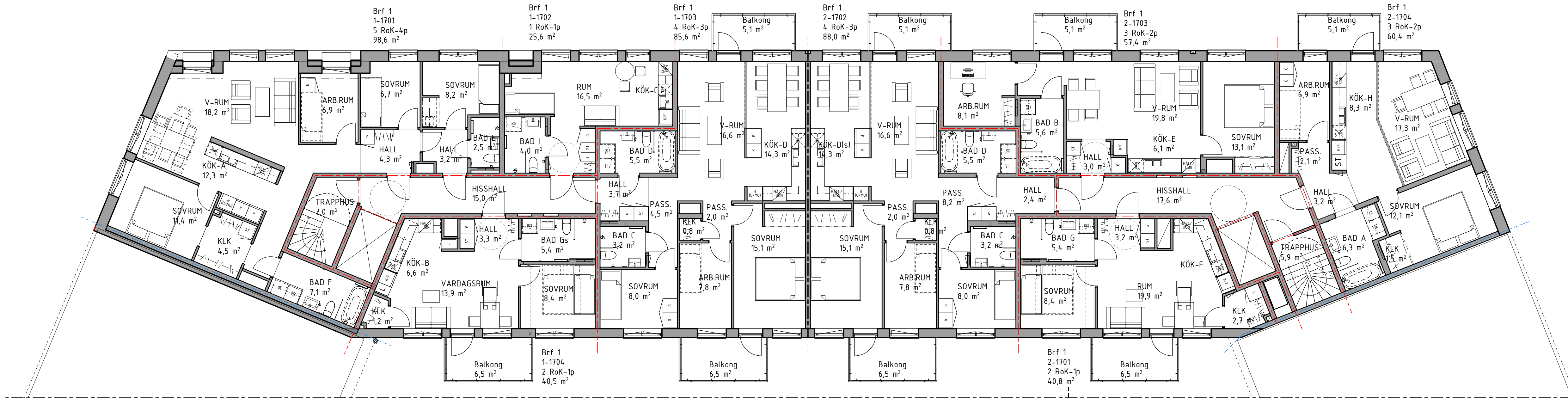
Plan 17 1:100
