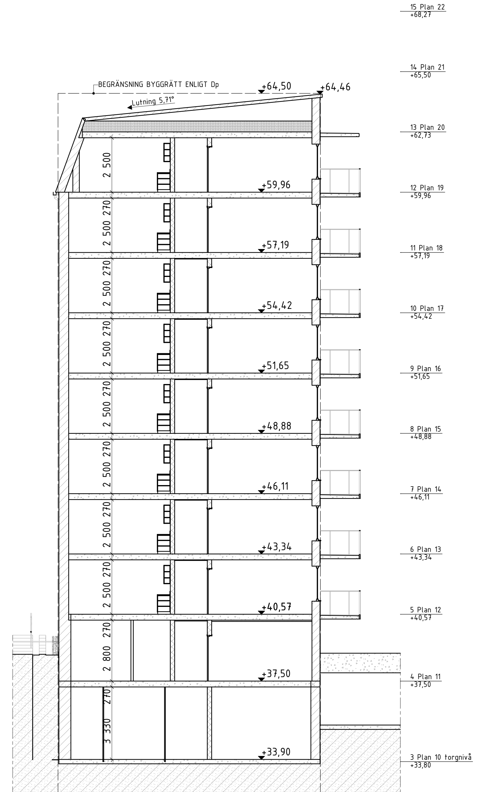
Tvärsektion 3 1:100
