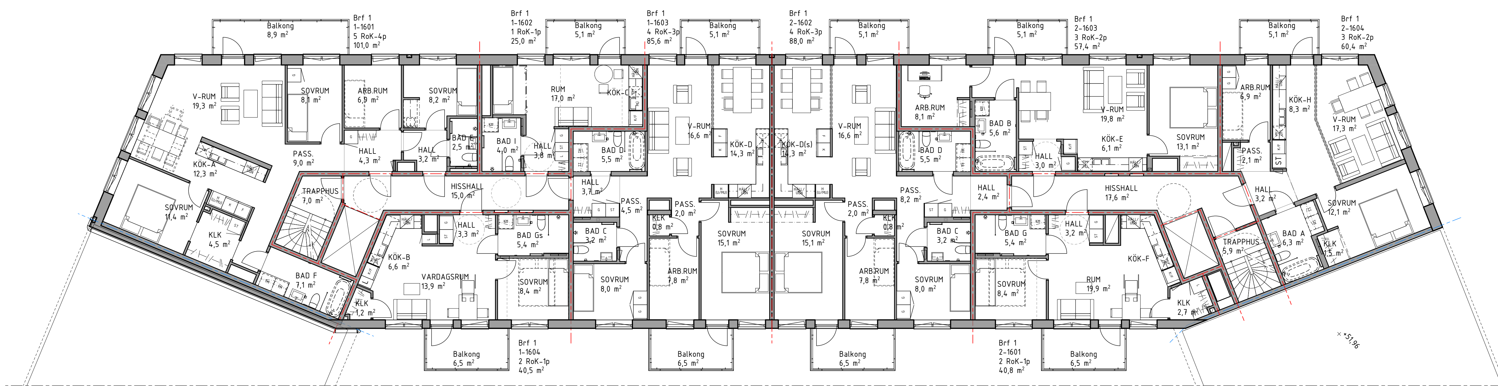
Plan 16 1:100
