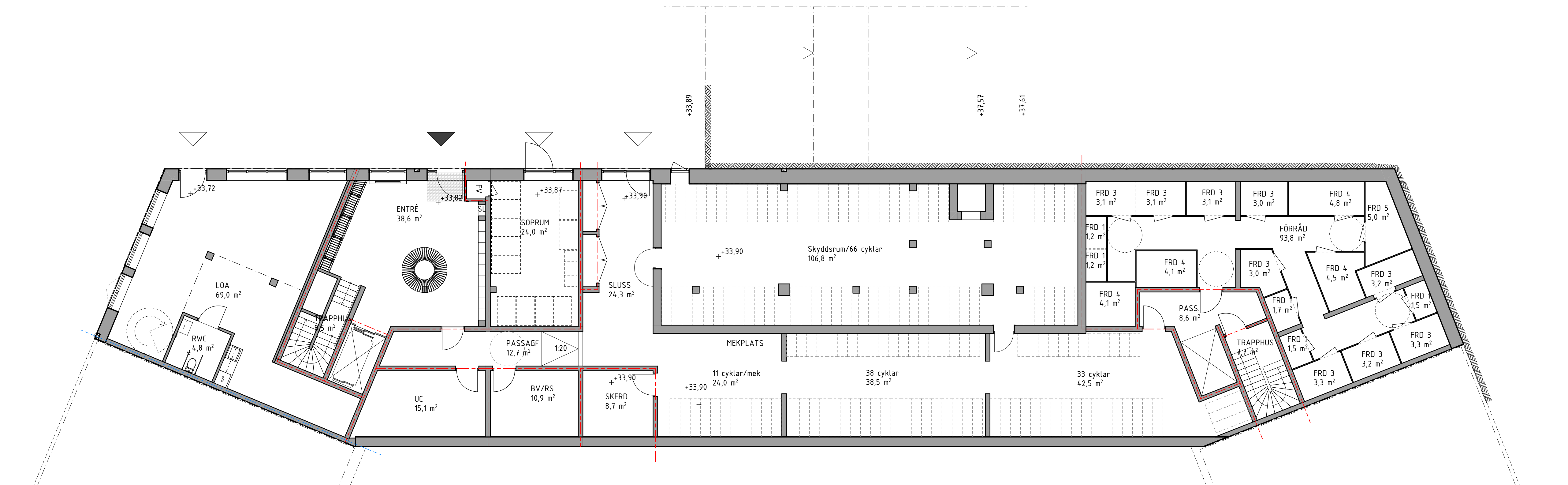
Plan 10 torgnivå 1:100
