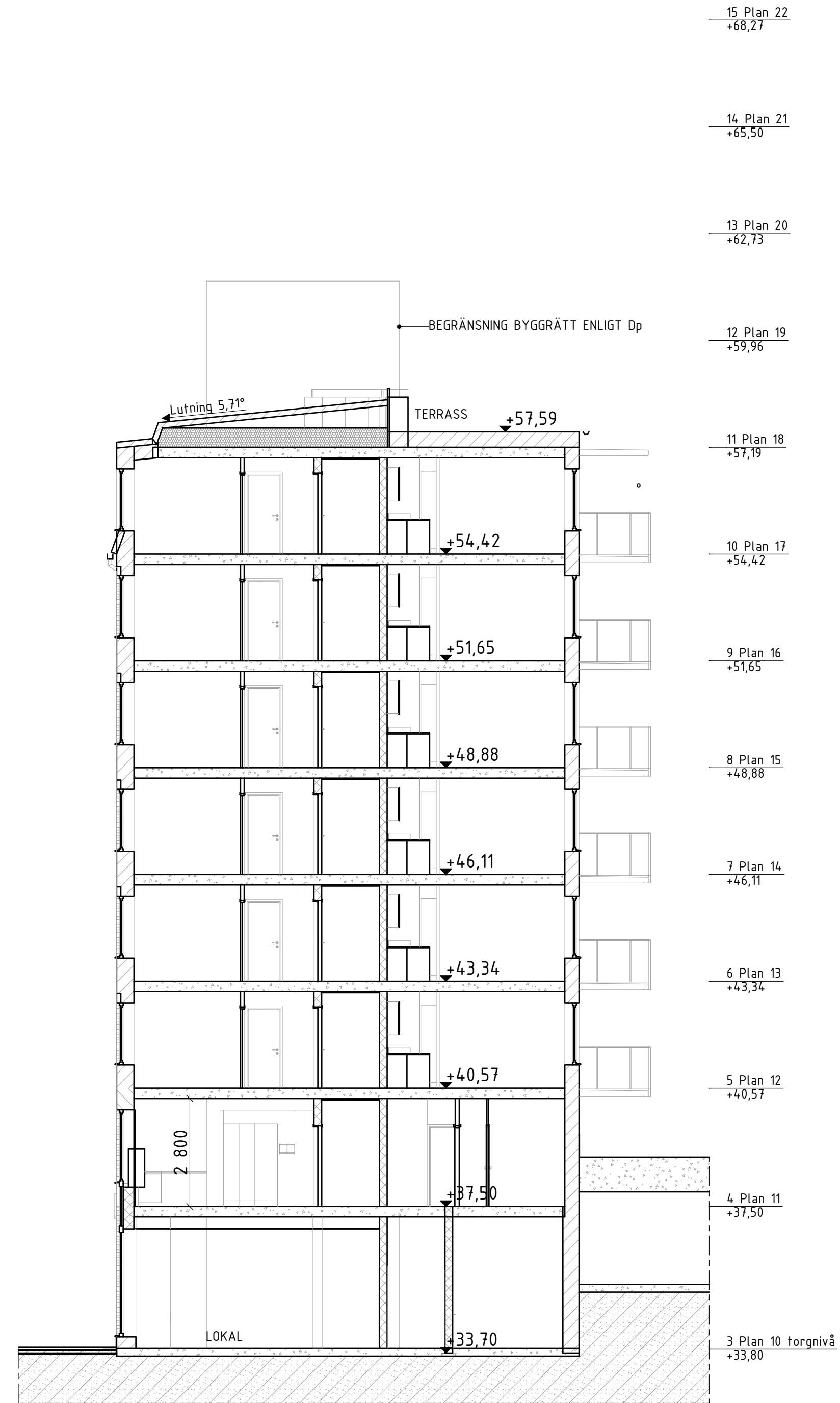
Tvärsektion 1 1:100
