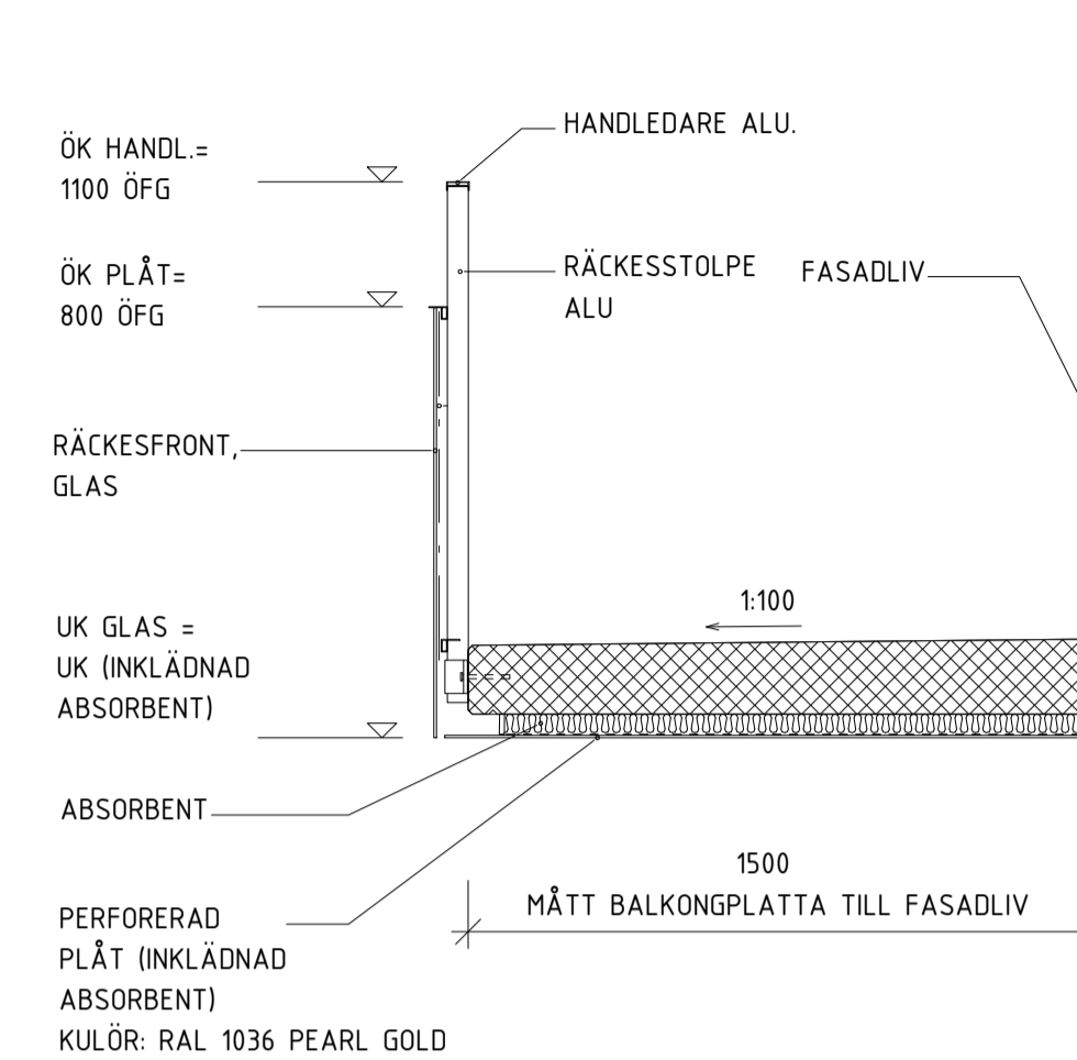
BALKONGPLATTOR MOT GATA, MED LJUDABSORBENT, SKALA 1:20
