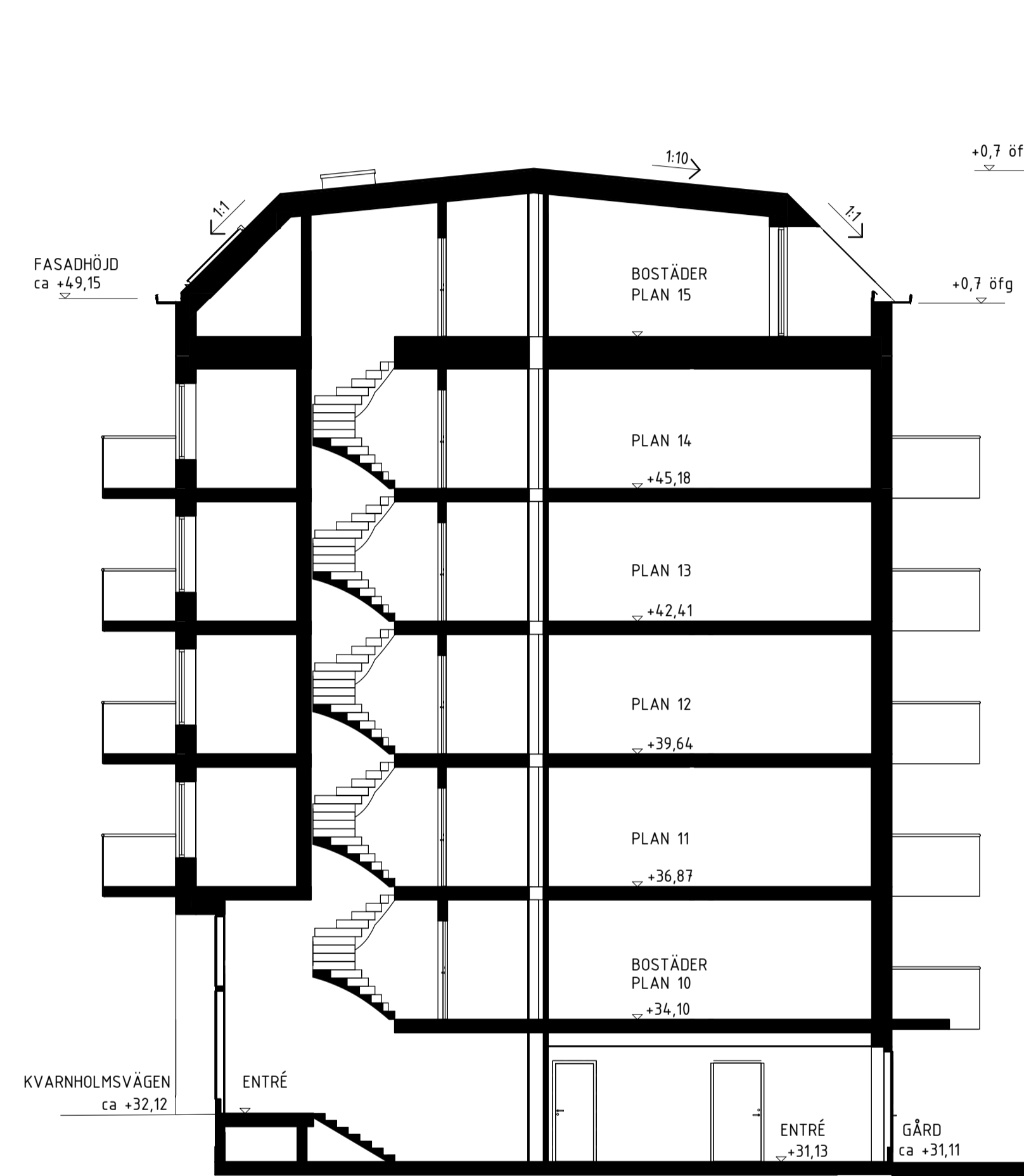
TVÄRSEKTION A-A, TH 2
