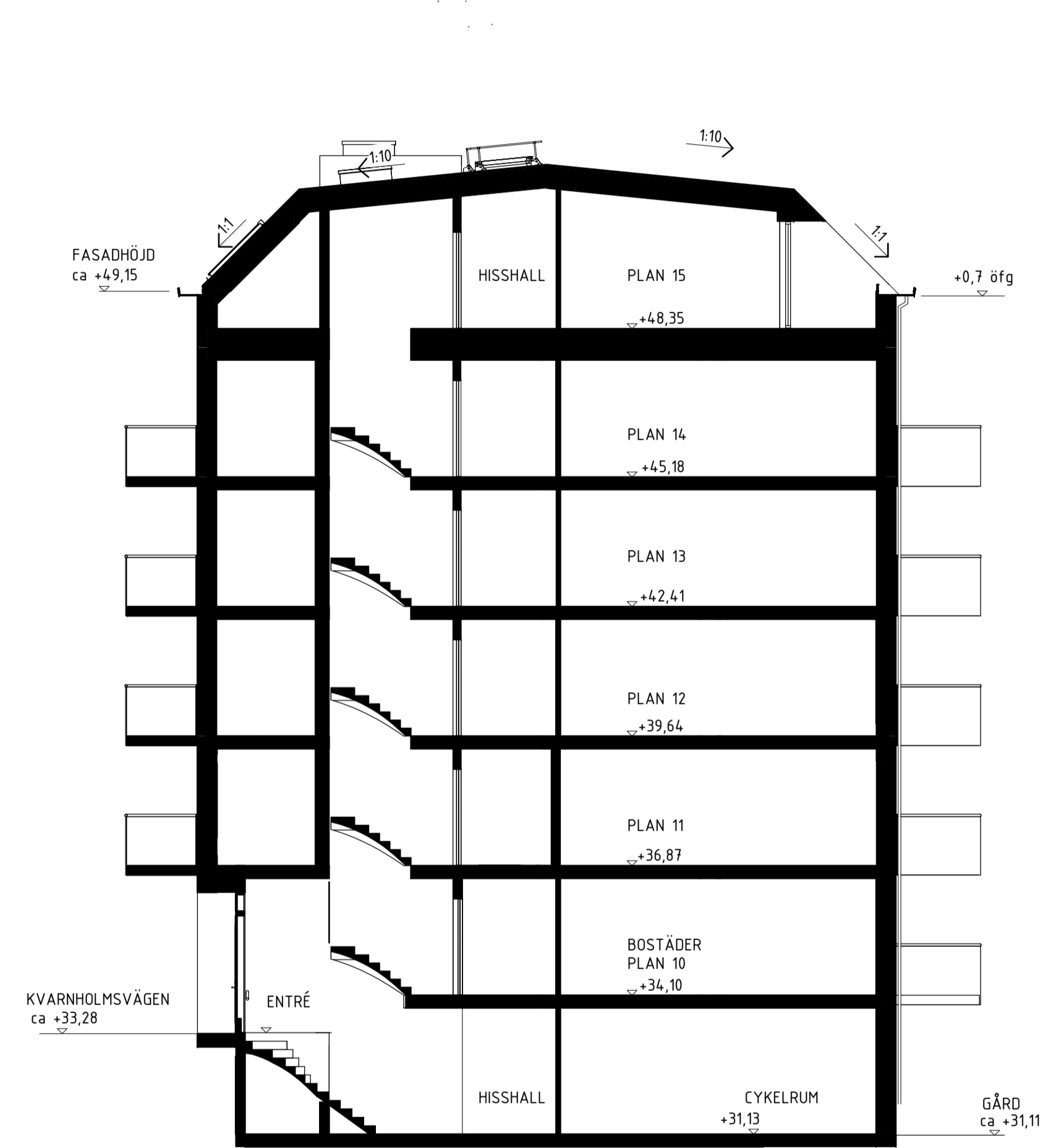
TVÄRSEKTION C-C, TH 4
