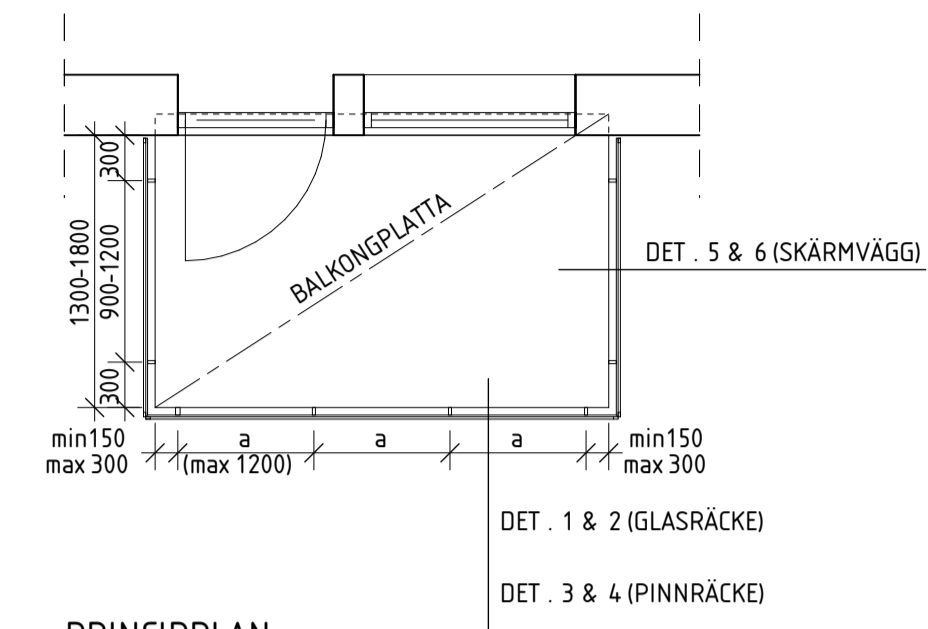
PRINCIPLAN 1:50
