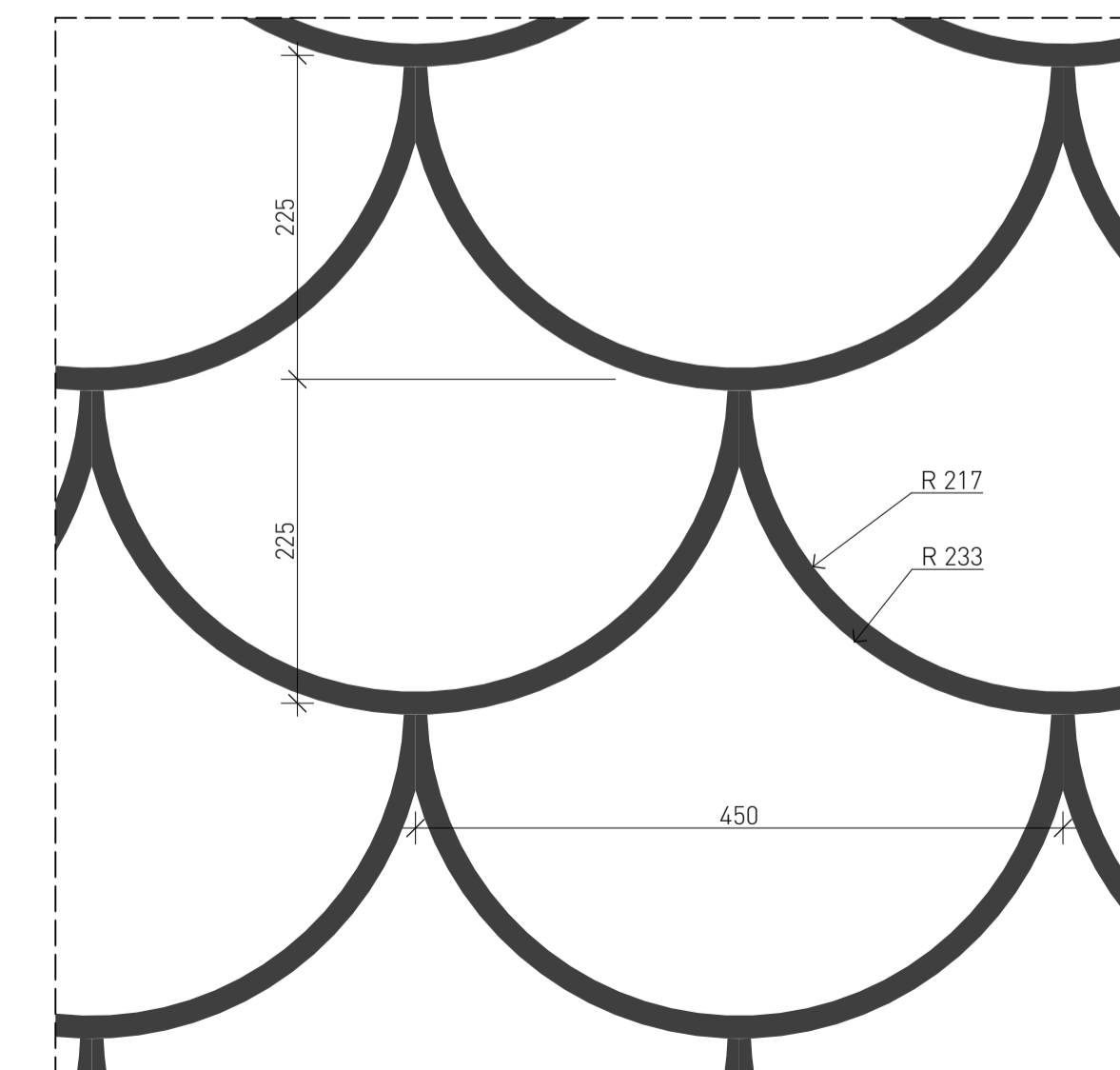
DET. 12 MÖNSTER I RÄCKE TYP C
