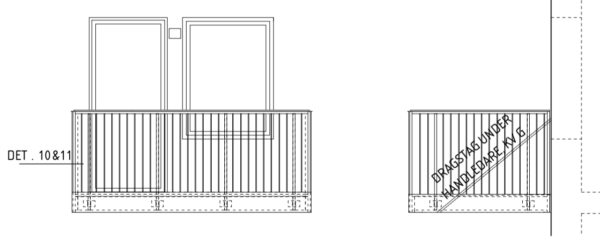
PRINCIPELEVATIONER BALKONG RÄCKE TYP B (PINNRÄCKE) 1:50
