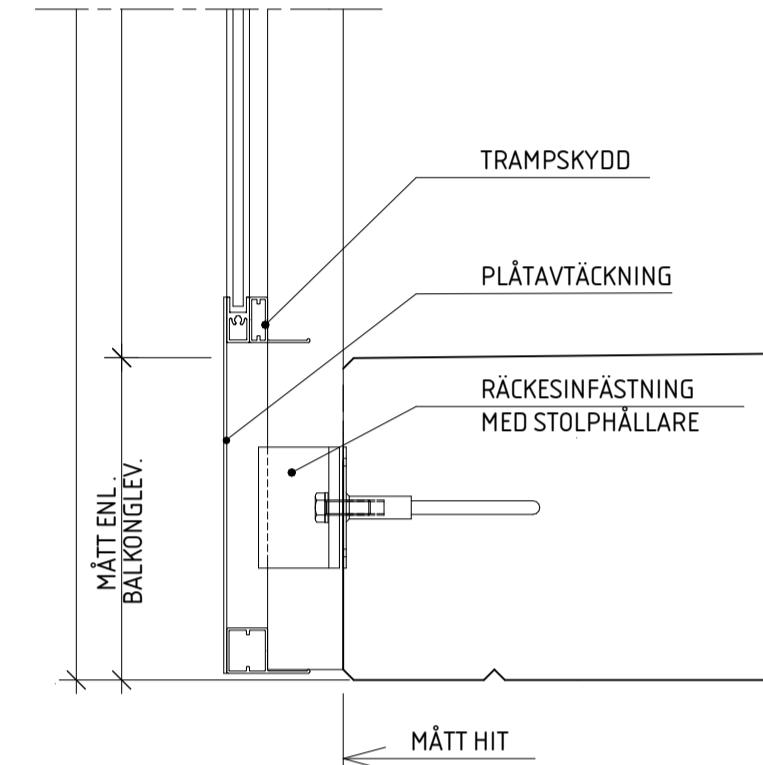
DET. 2 VERTIKALSNIITT INFÄSTNING MOT BALKONGPLATTA 1:5
