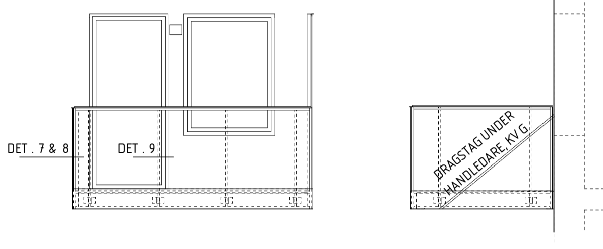
PRINCIPELEVATIONER BALKONGRÄCKE TYP A (GLASRÄCKE) 1:50
