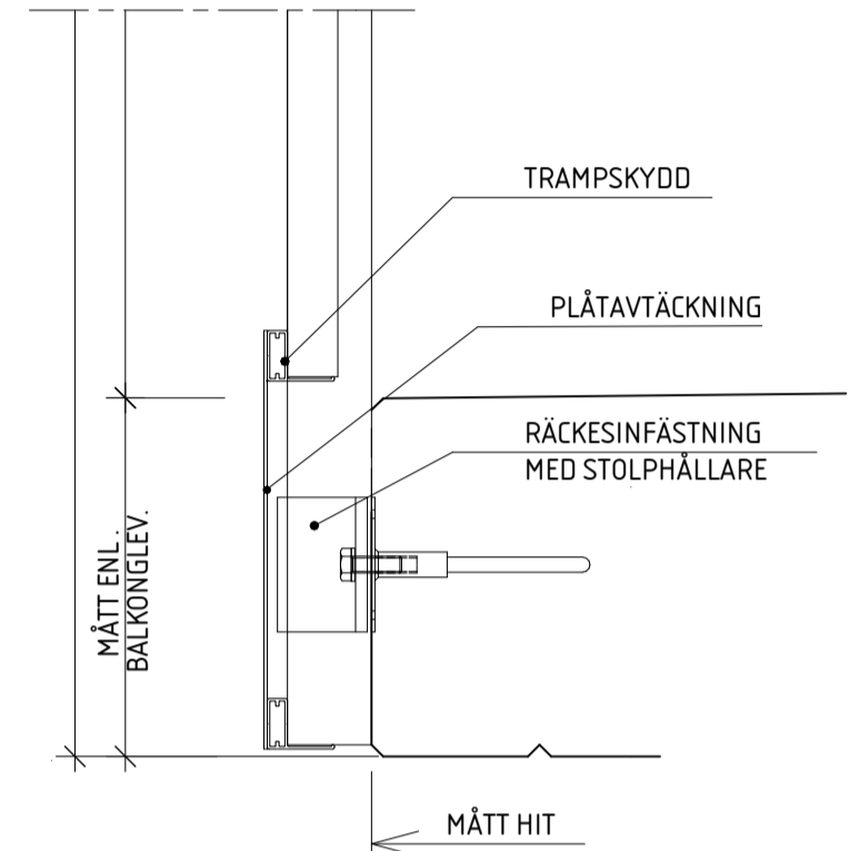
DET. 4 VERTIKALSNIITT INFÄSTNING MOT BALKONGPLATTA 1:5
