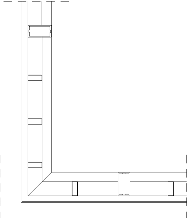
DET. 11 HORIZONTALSNIITT YTTERHÖRN PINNRÄCKE 1:5
