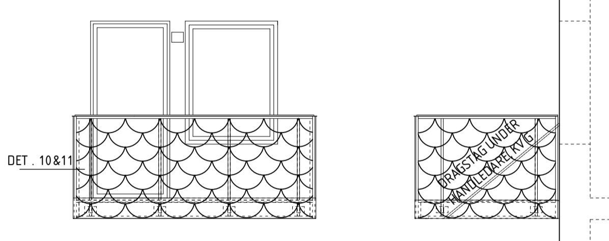
PRINCIPELEVATIONER BALKONG RÄCKE TYP C (GLASRÄCKE MÖNSTRAT) 1:50
