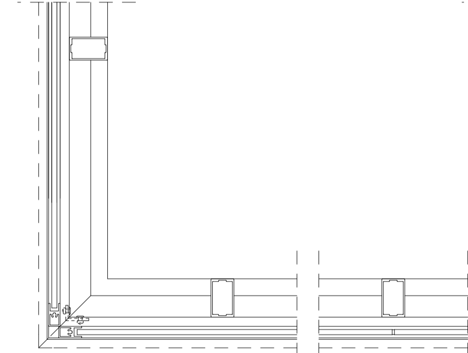
DET. 8 HORIZONTALSNIITT YTTERHÖRN GLASRÄCKE 1:5
