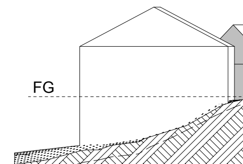
Hus C Fasad mot norr 1:200
