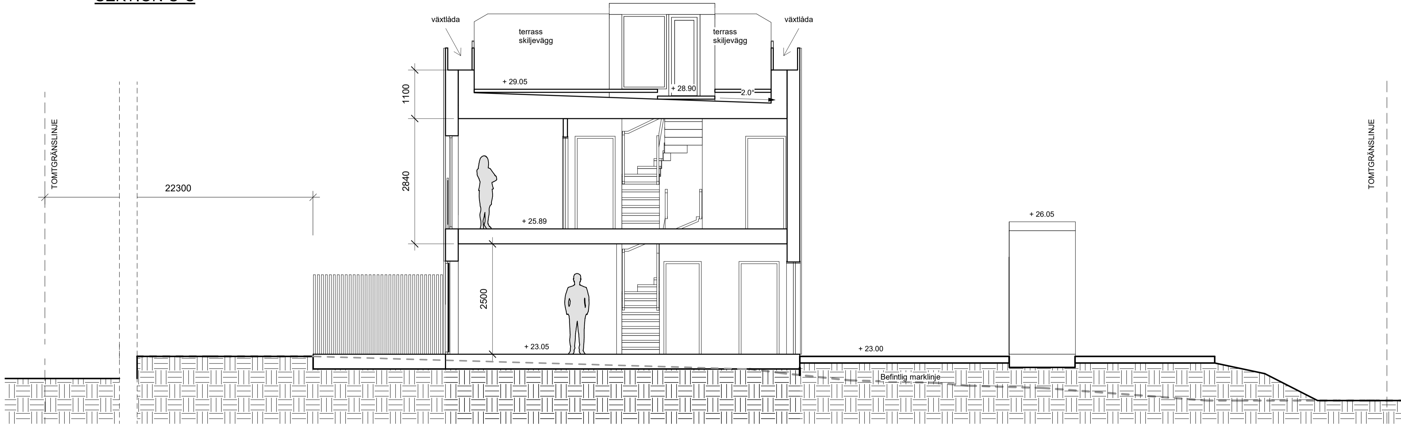
SEKTION C-C
