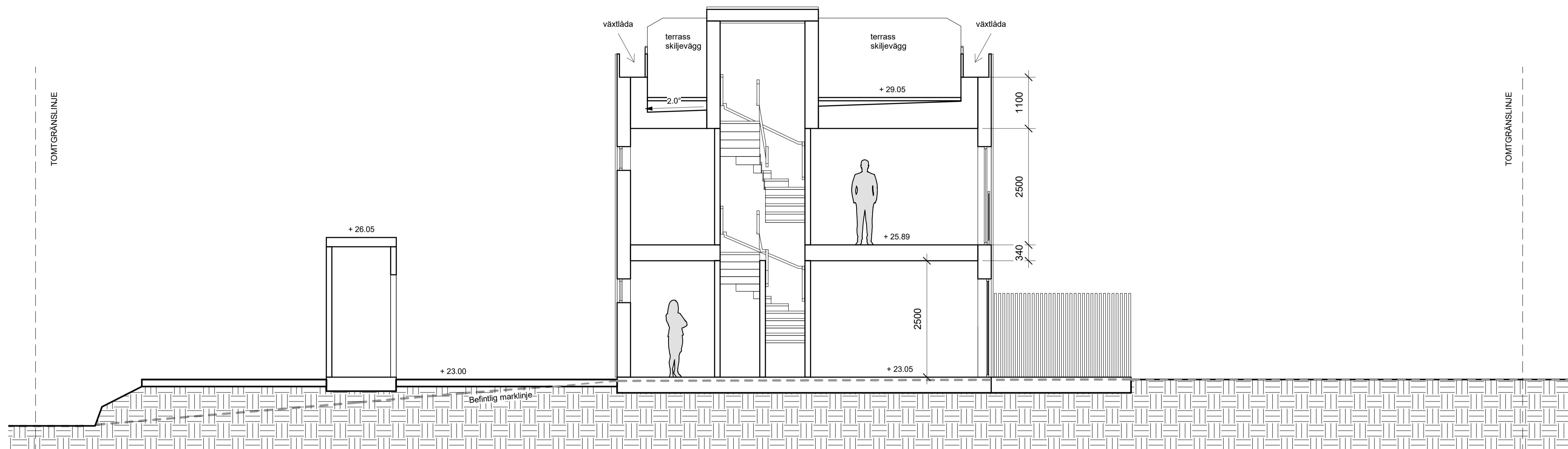
SEKTION A-A
