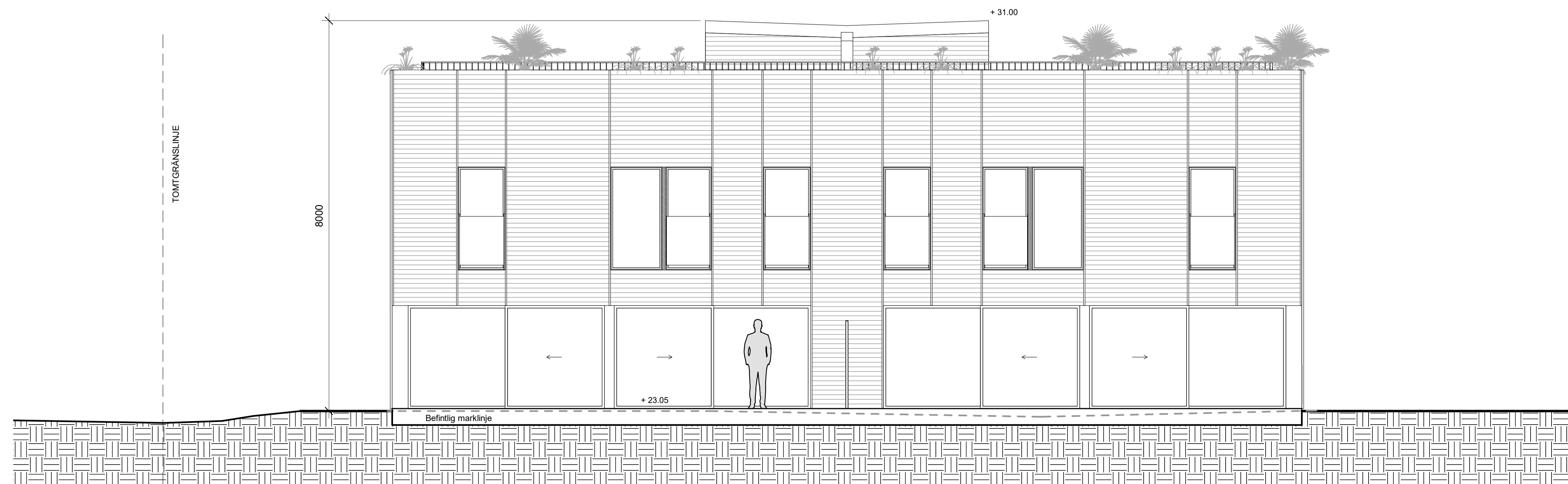
FASAD SYDVÄST
