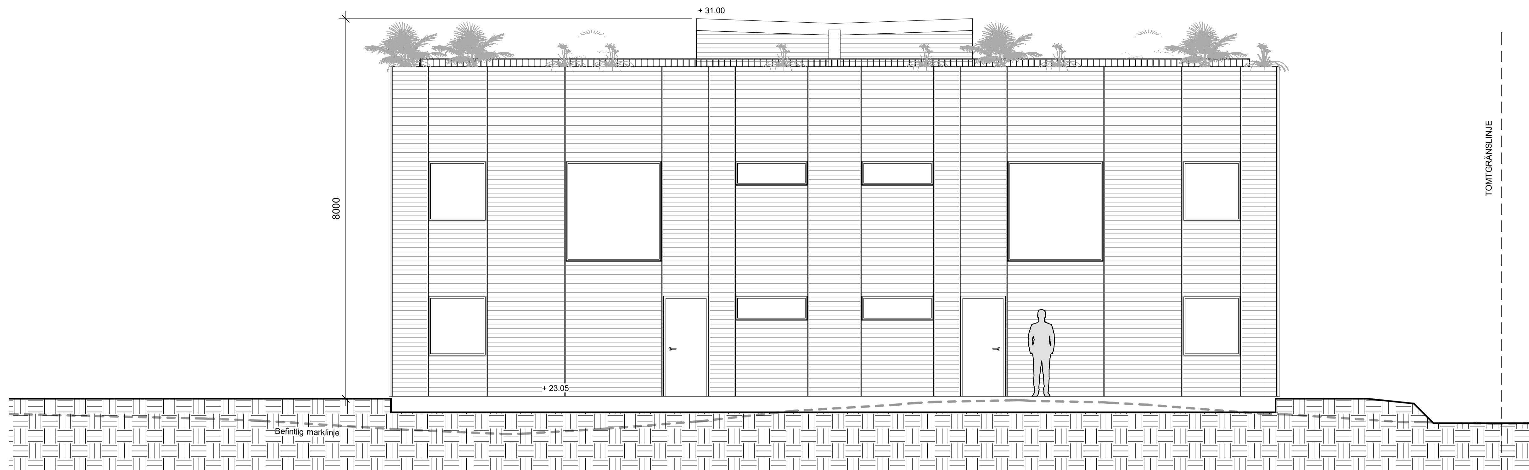
FASAD NORDOST
