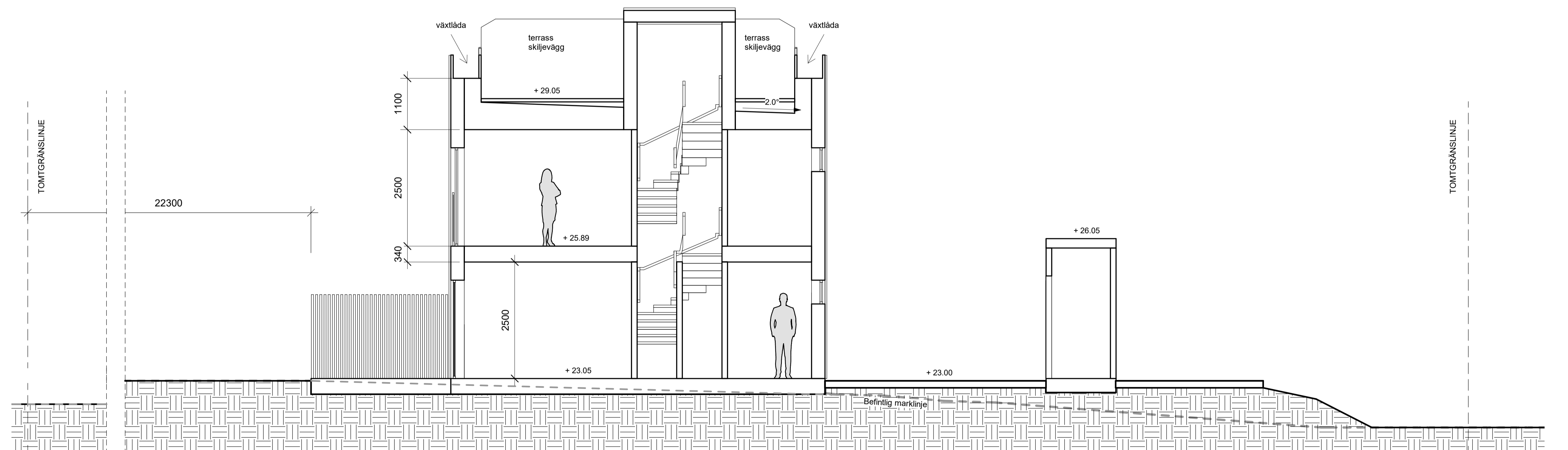
SEKTION B-B
