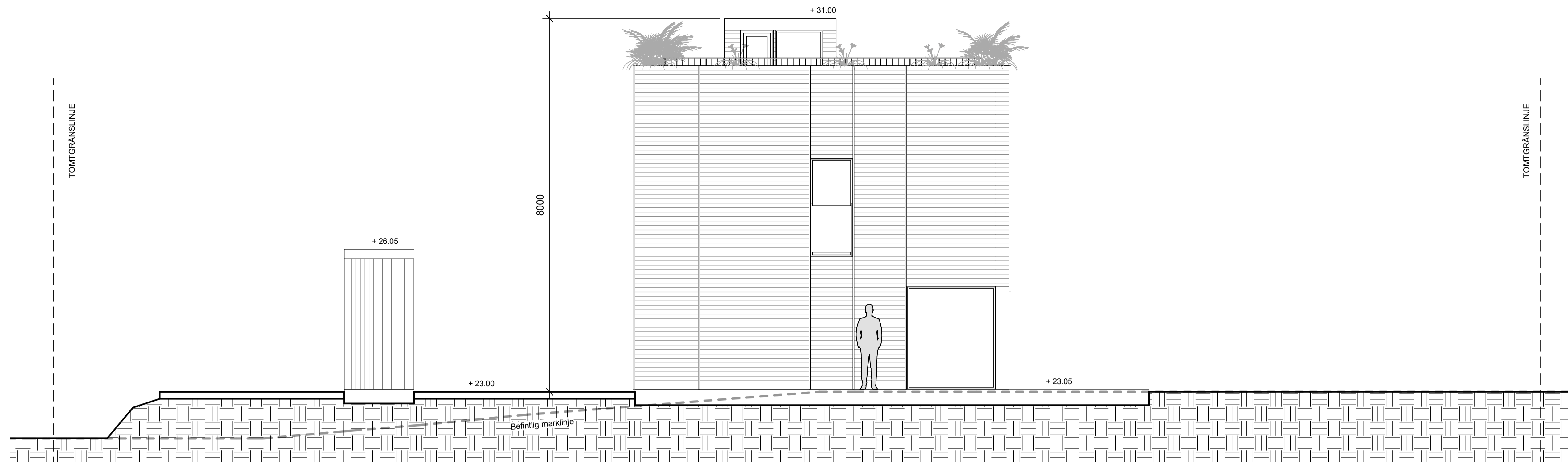
FASAD NORDVÄST
