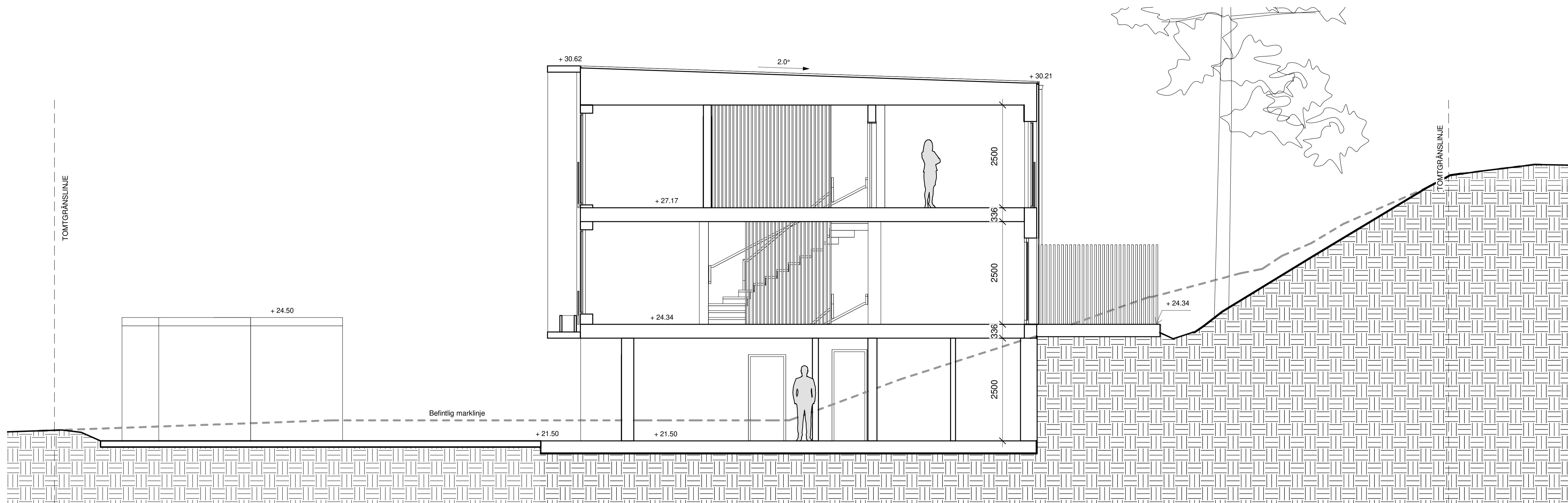
SEKTION B-B
