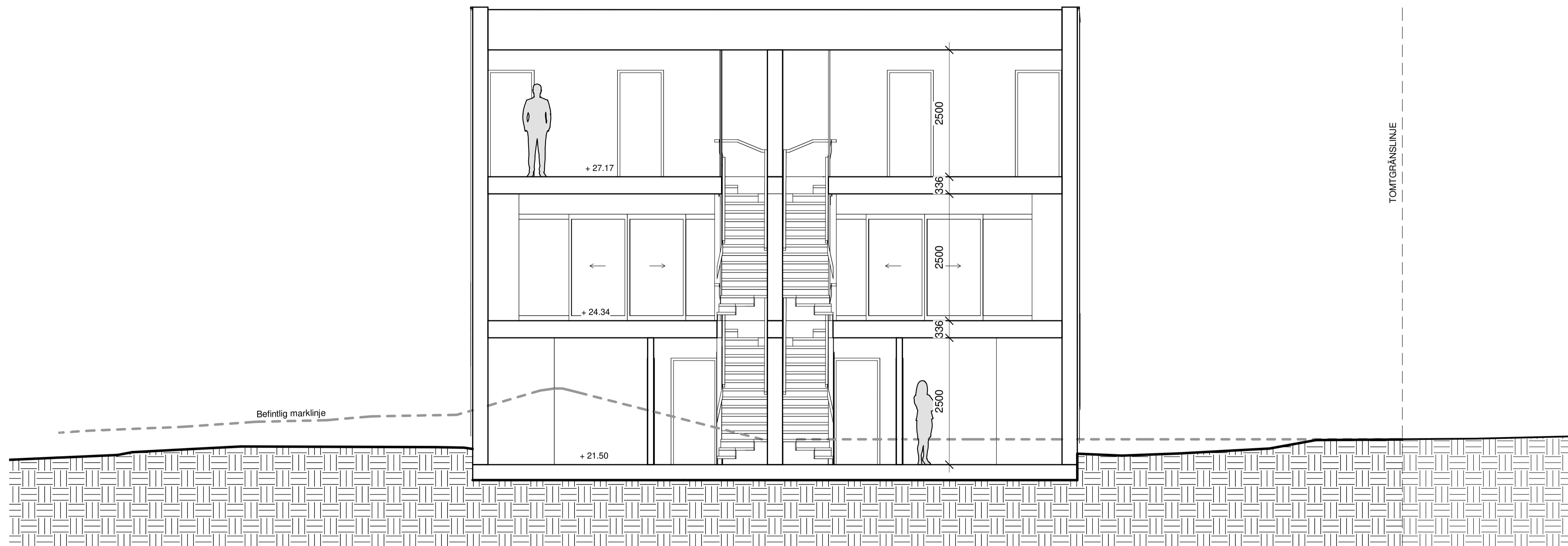
SEKTION A-A
