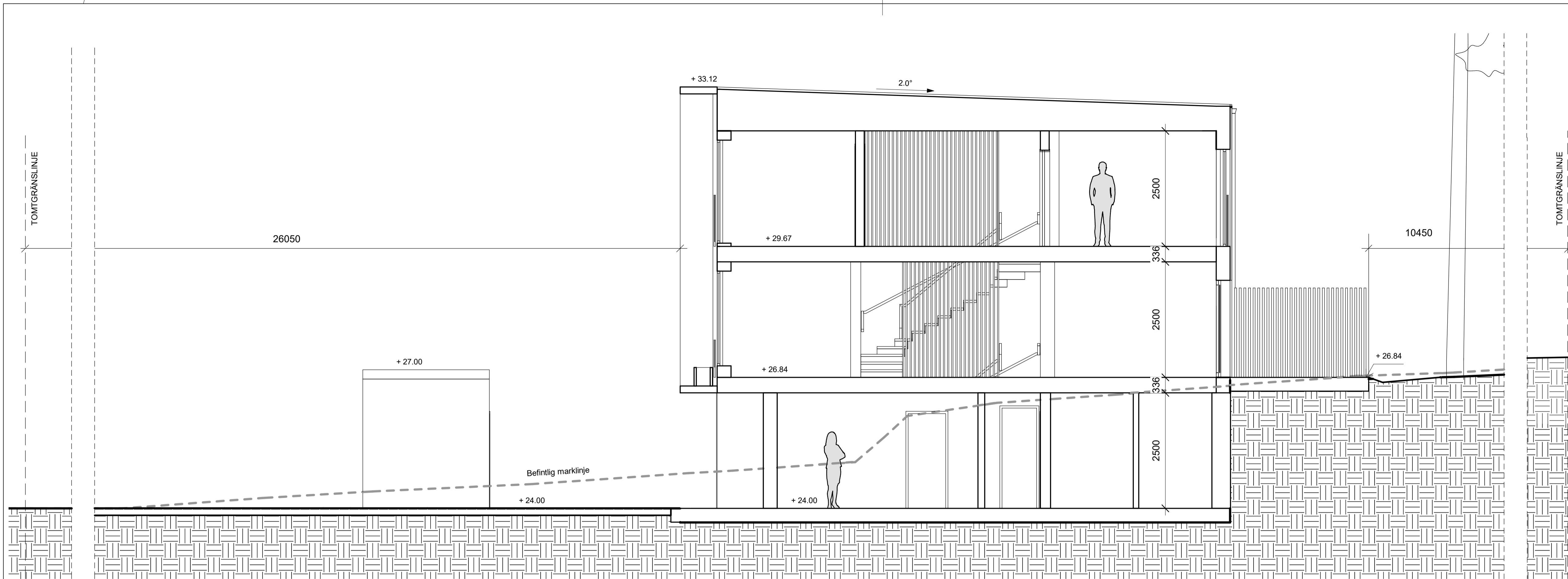
SEKTION B-B
