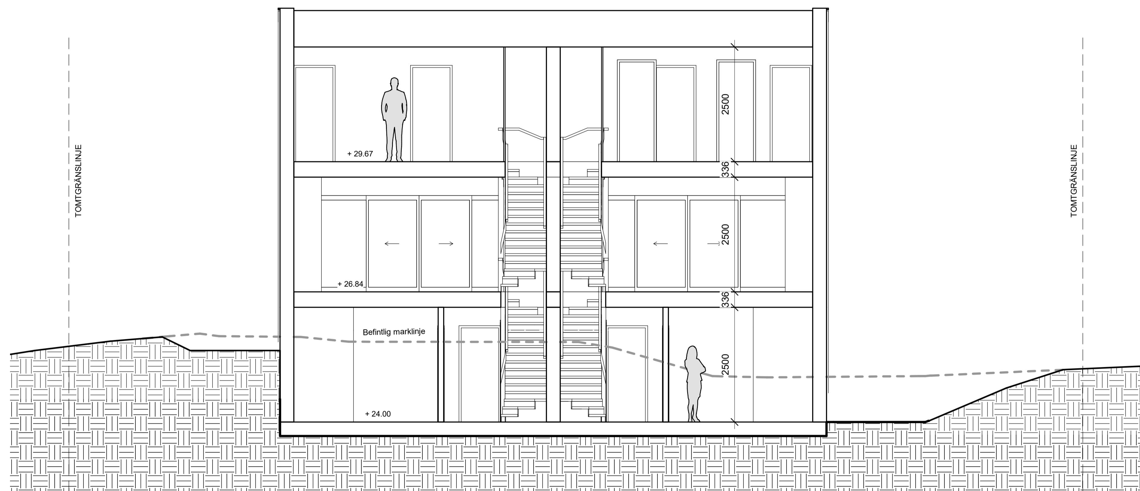
SEKTION A-A
