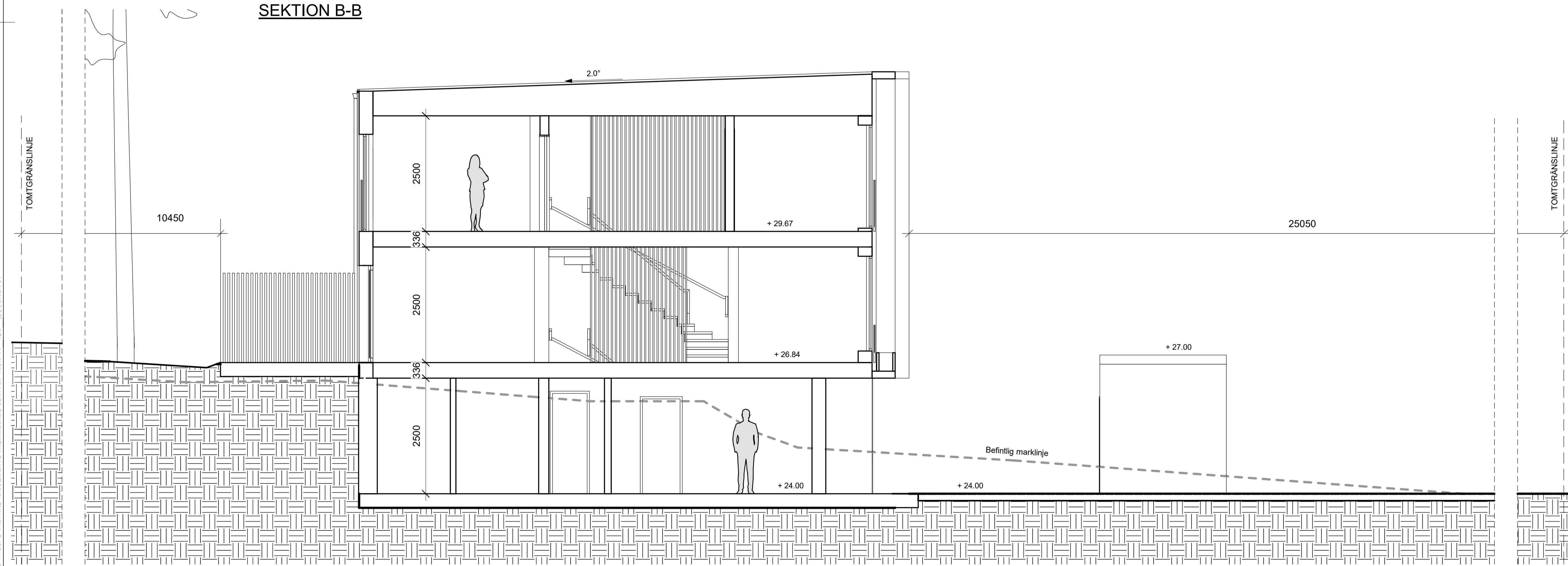
SEKTION C-C
