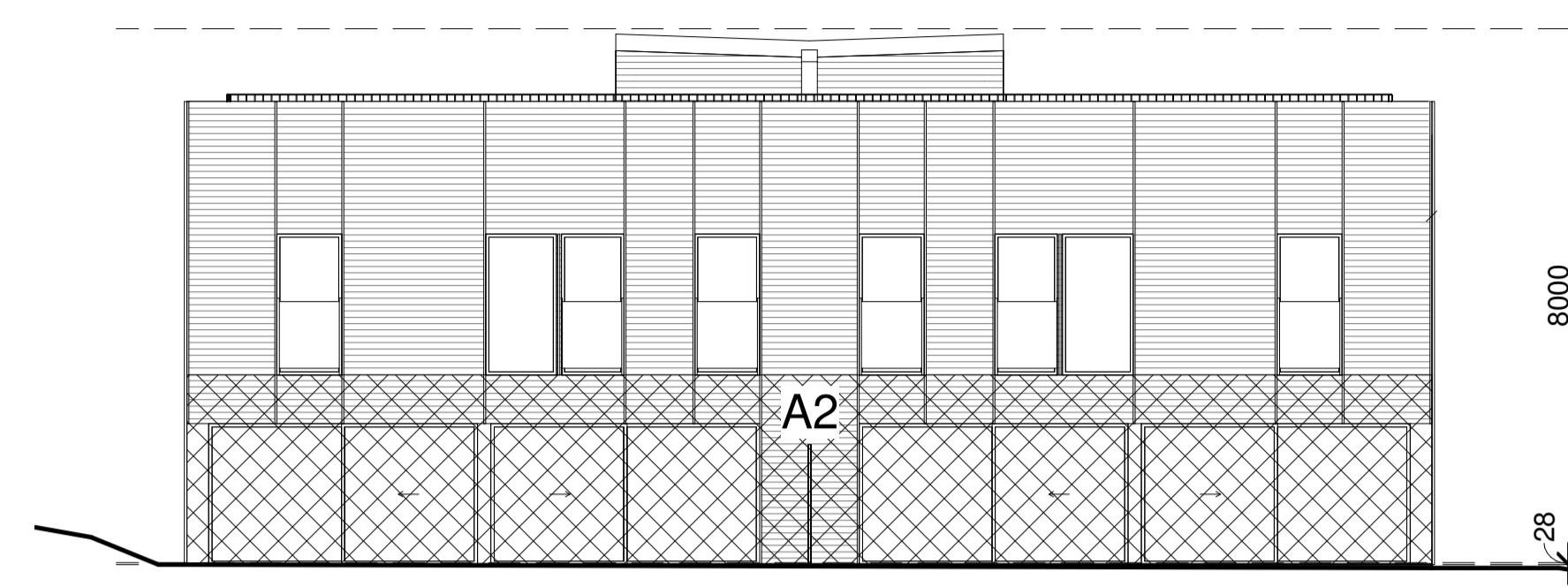
FASAD NORDVÄST
