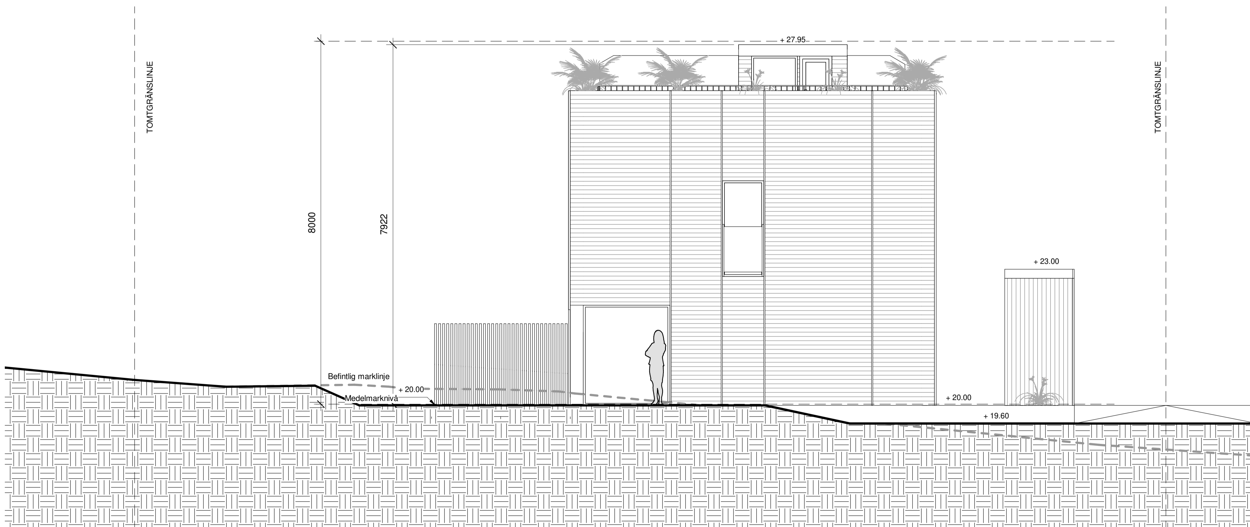
FASAD NORDOST
