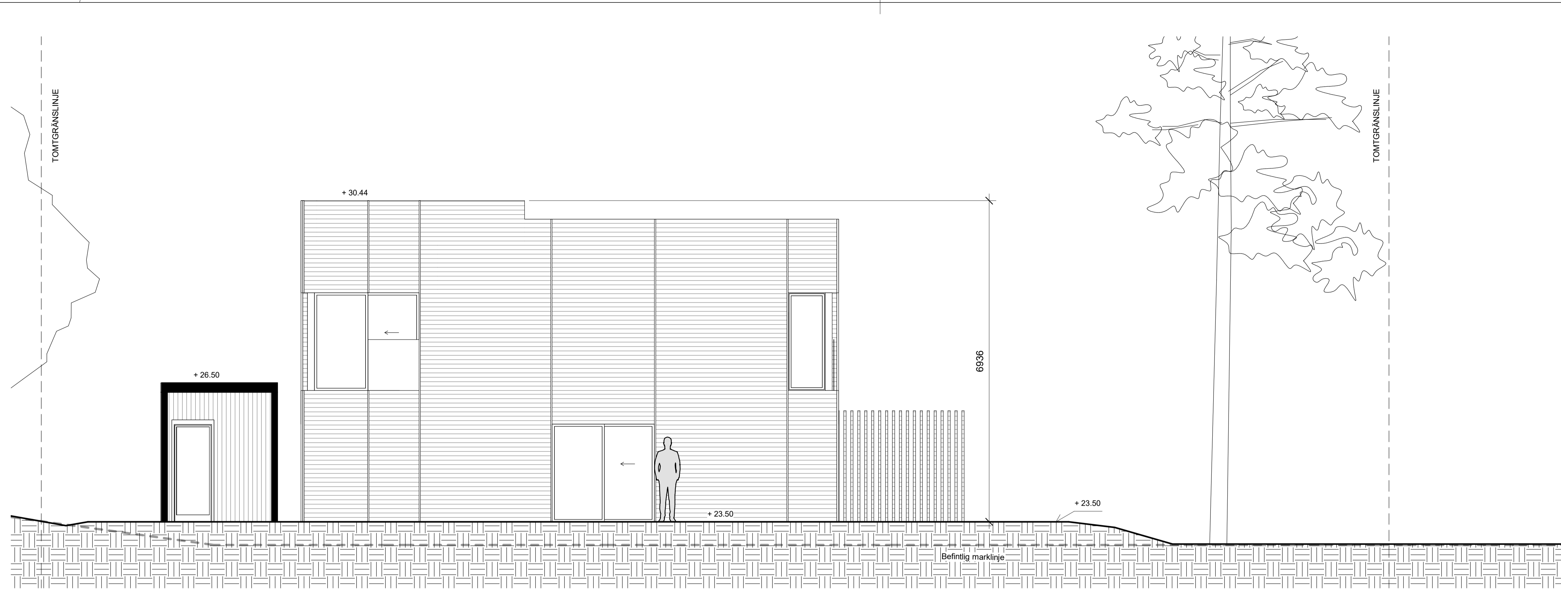
FASAD NORR
