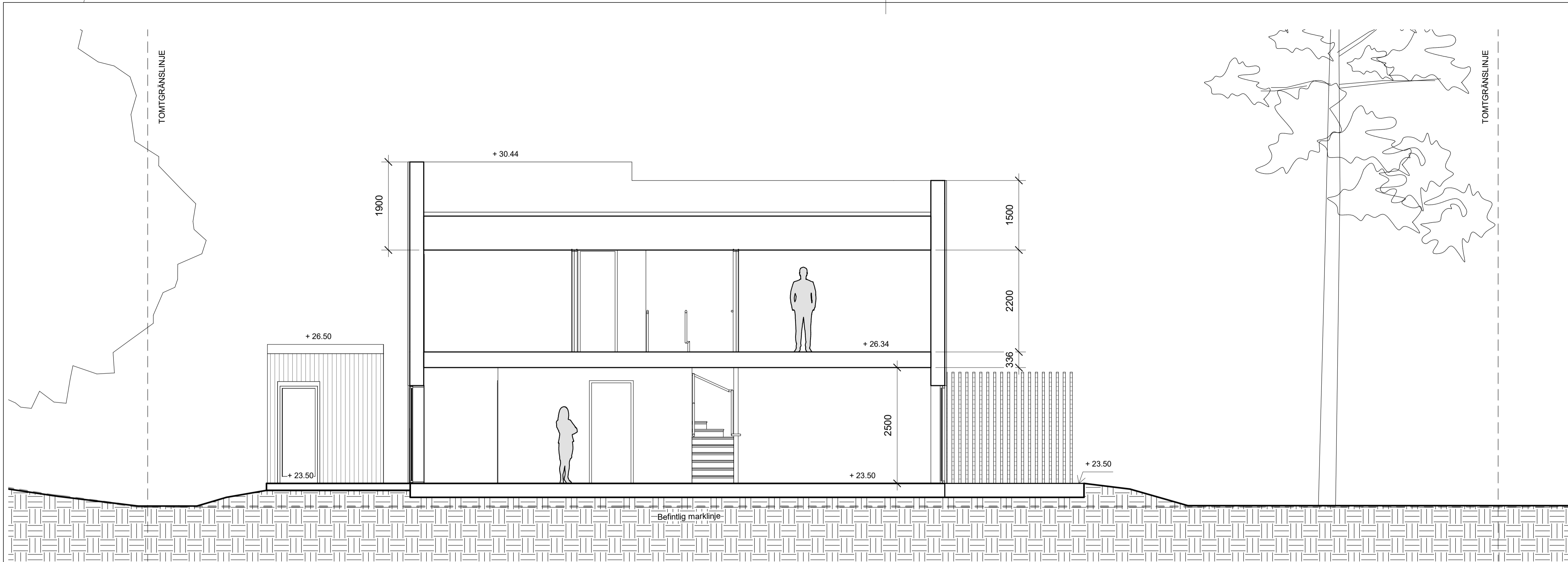
SEKTION B-B
