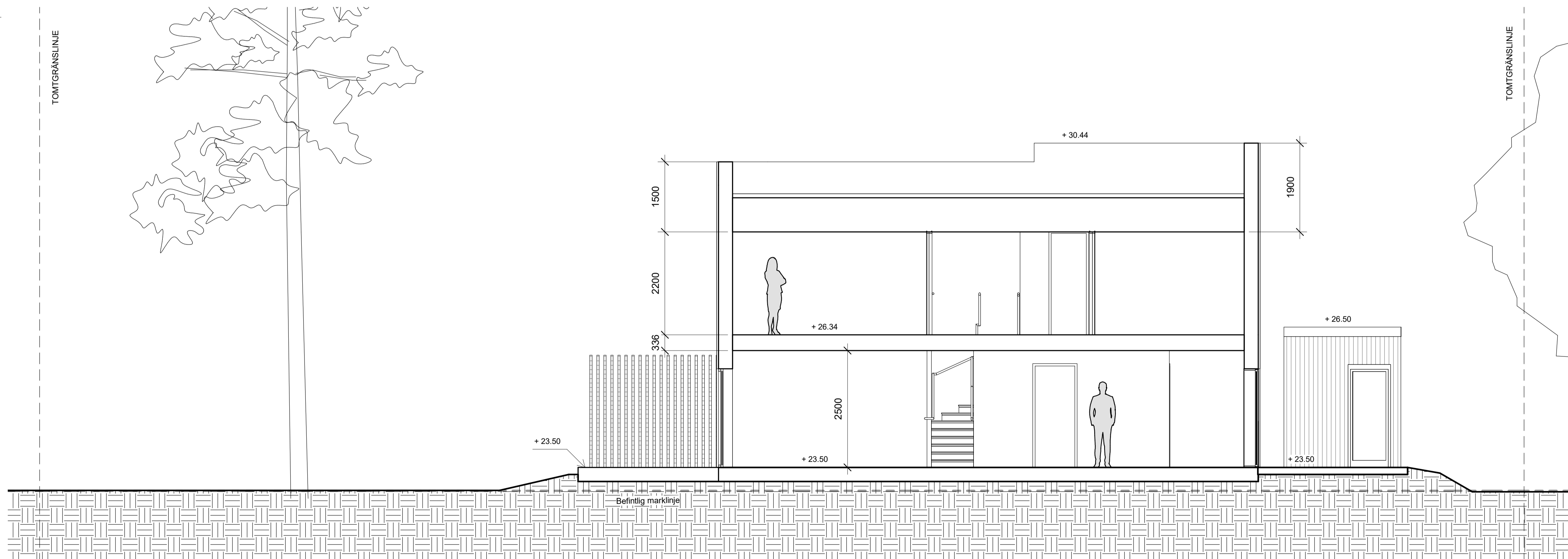
SEKTION B-B
