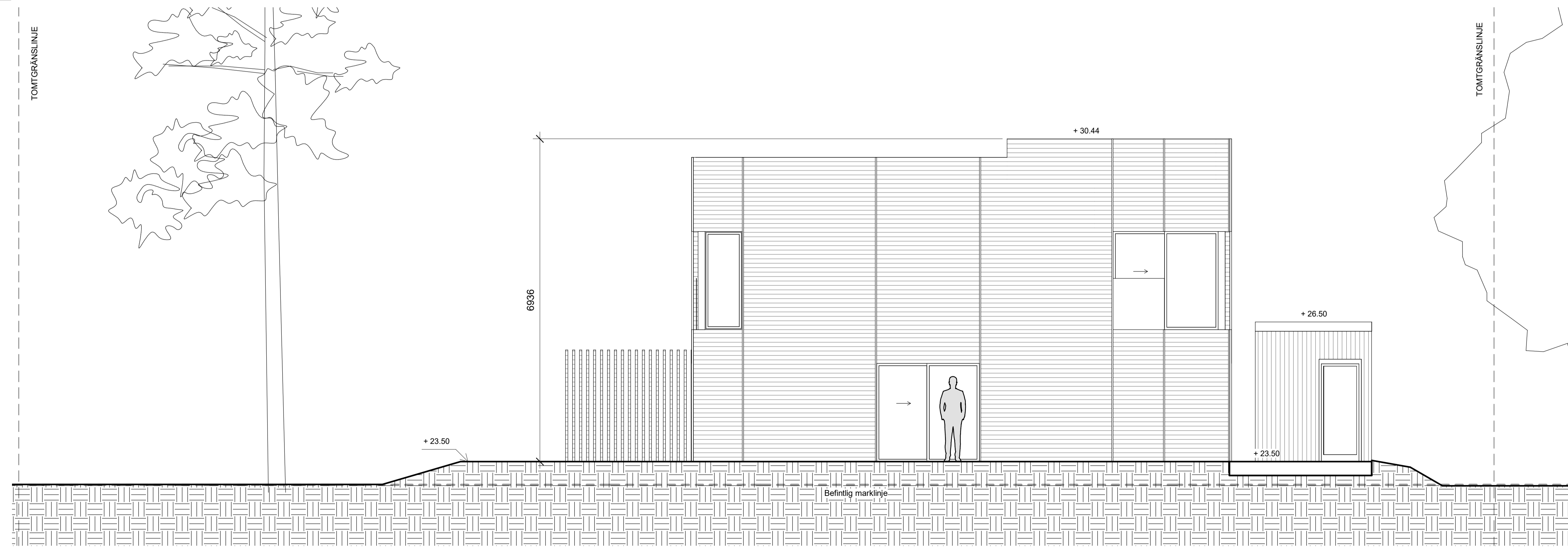
FASAD SÖDER
