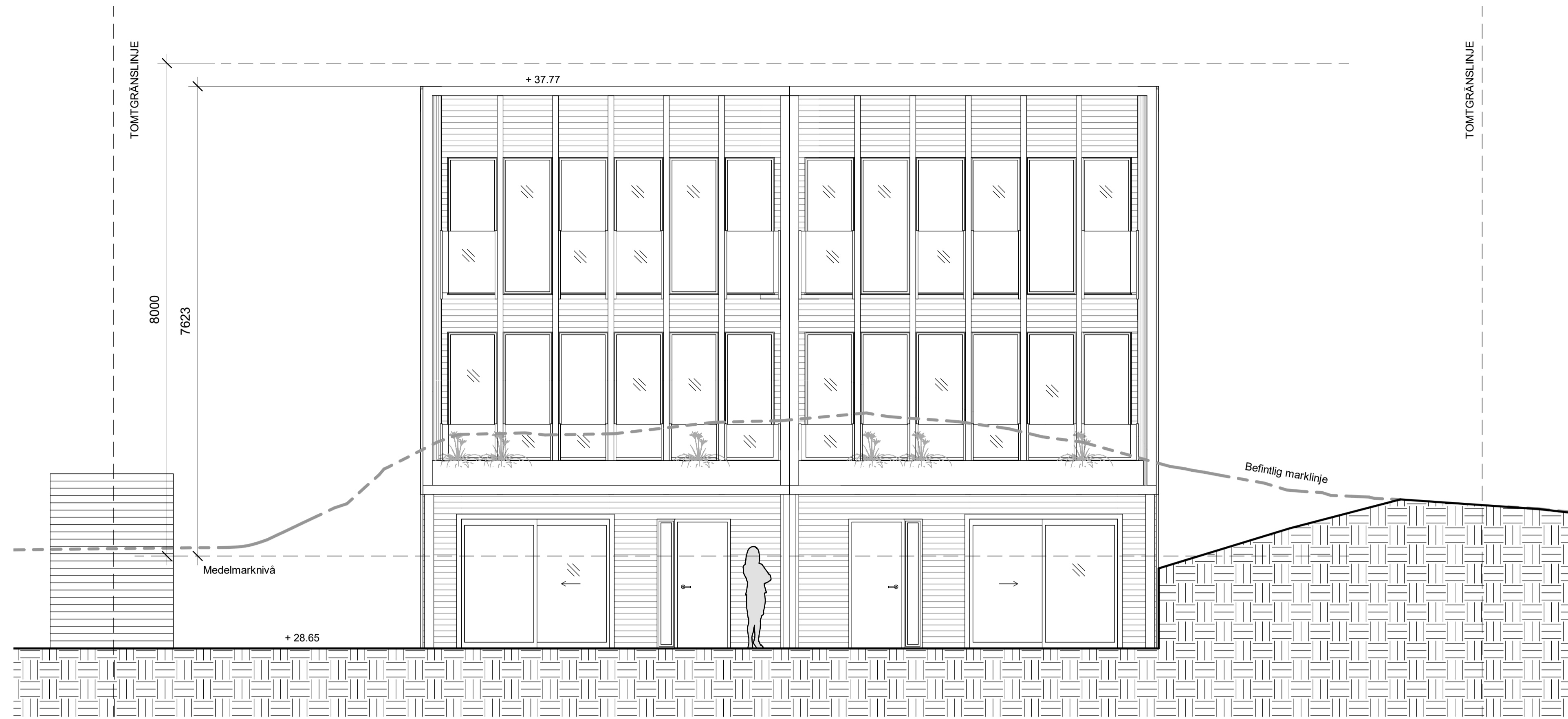
FASAD SYDVÄST
