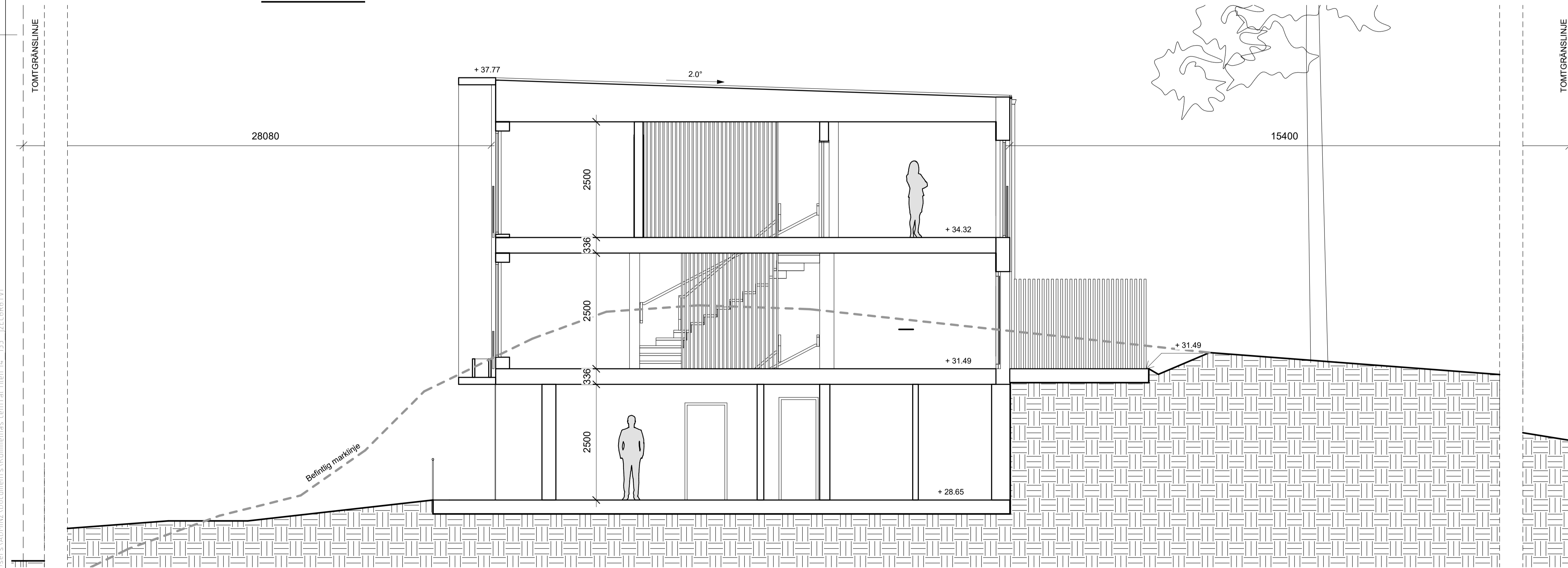
SEKTION B-B
