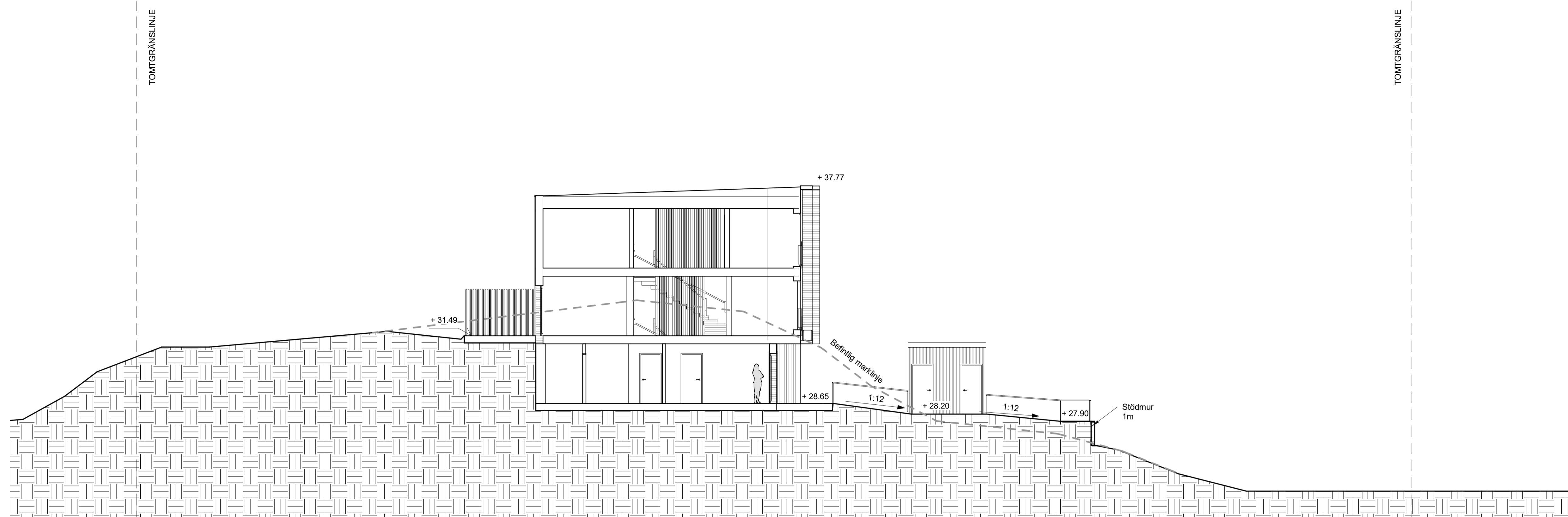
SEKTION D-D
