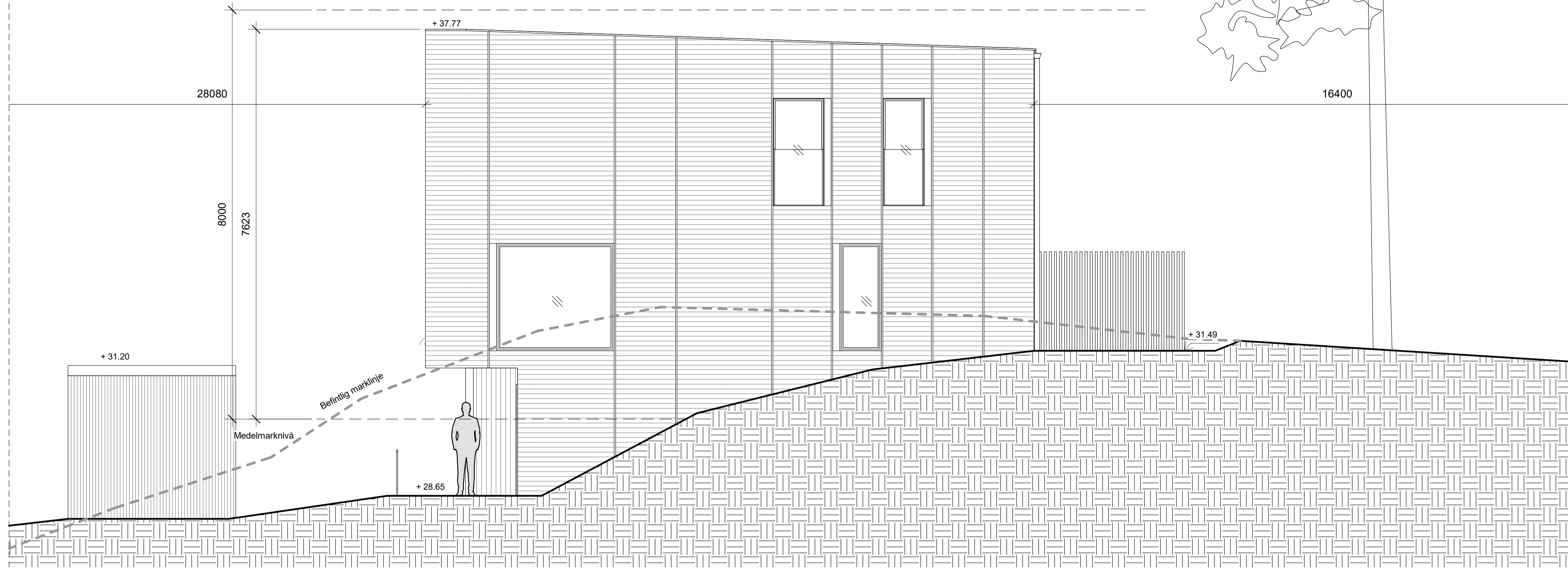
FASAD SYDOST
