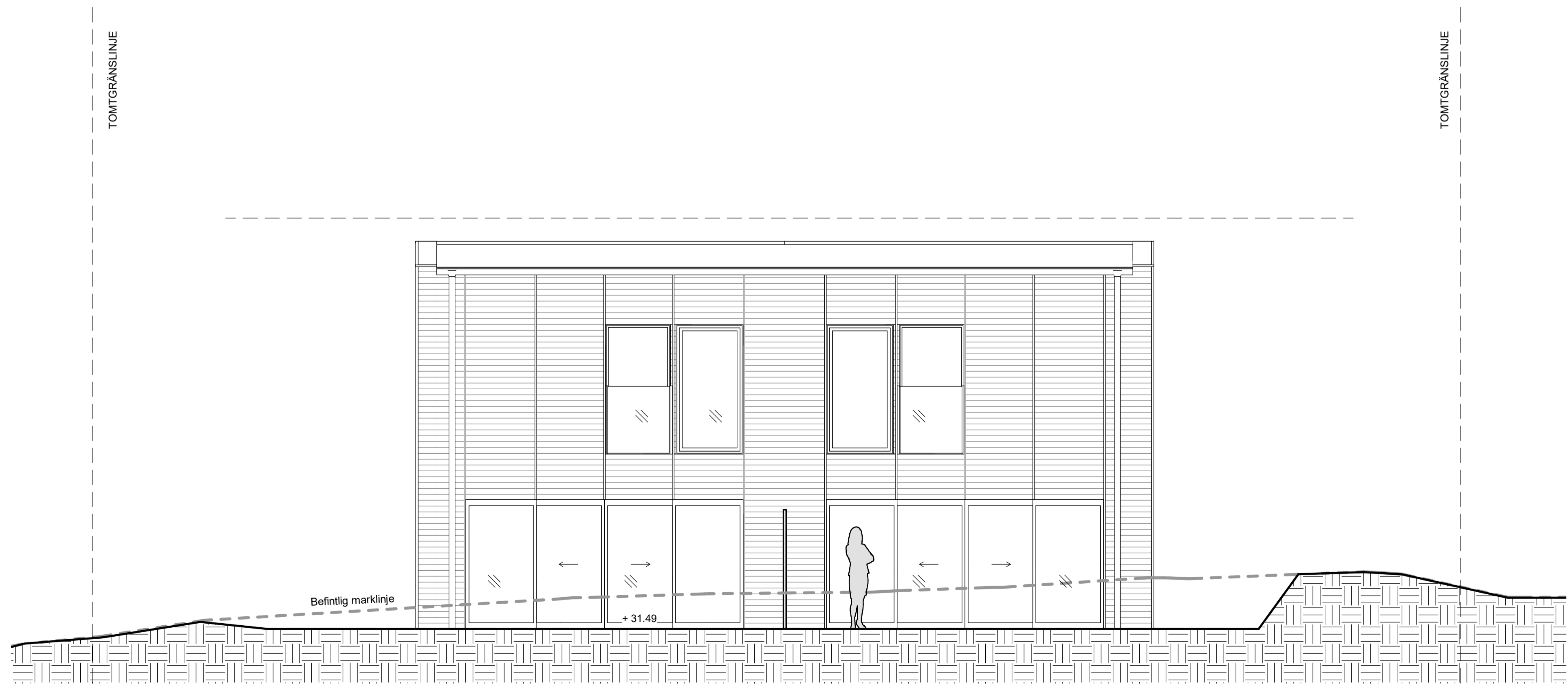
FASAD NORDOST
