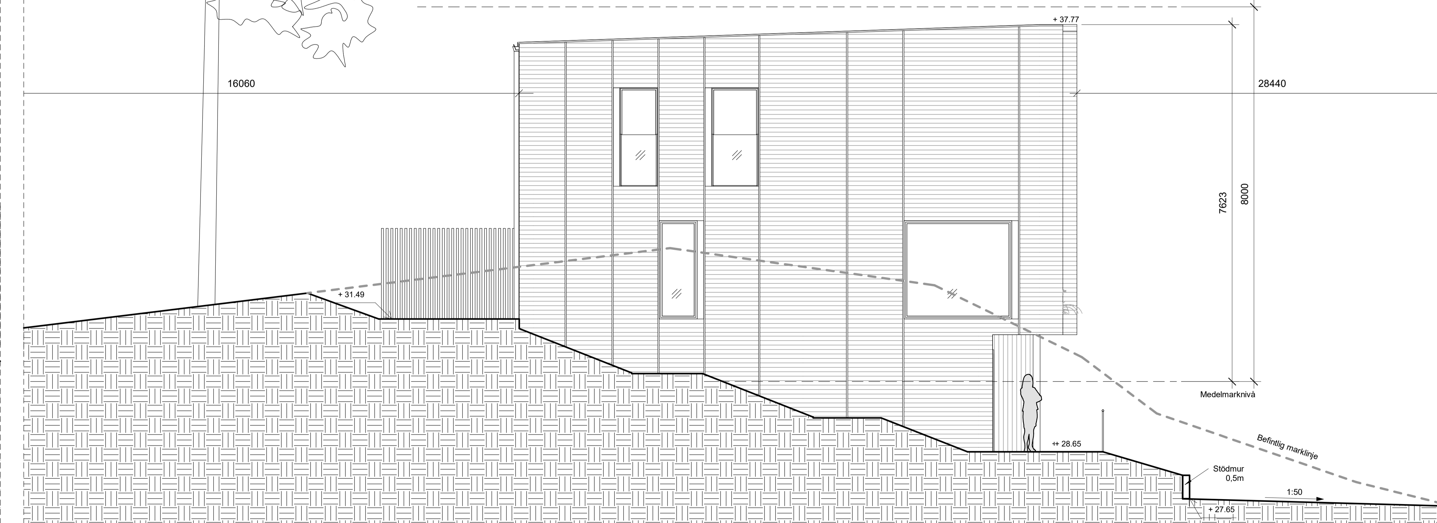
FASAD NORDVÄST
