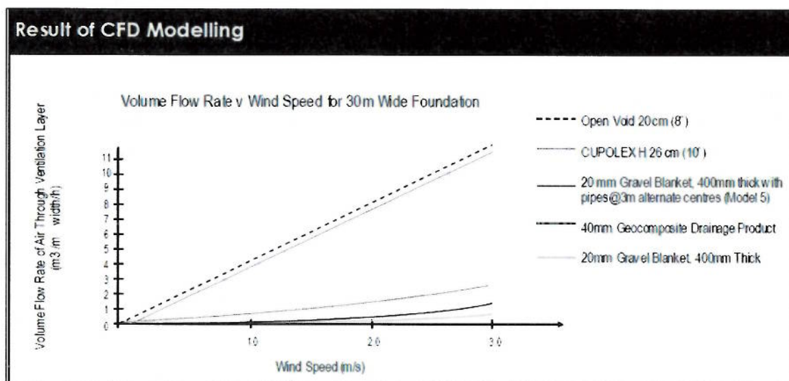
Figur 11. Jämförelse av luftflöden genom Cupolex® hålvolym jämfört med dräneringsprodukter av grus och geokomposit. Efter Ove Arup, 1997.
