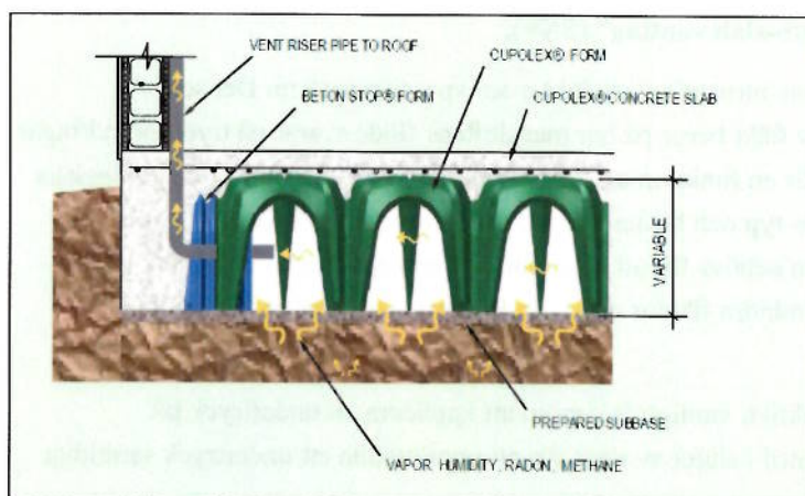
Figur 9. Cupolex® ventilerat golvsystem. Från Pontarolo Engineering, Inc.
