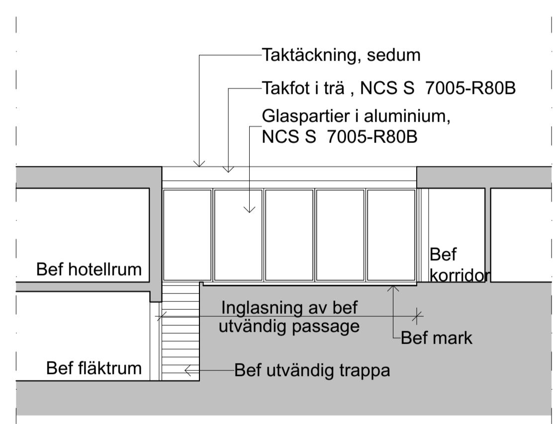
VY 4 Fasad mot väster
