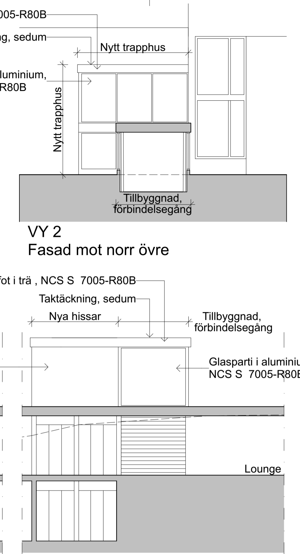
VY 2 Fasad mot norr övre
