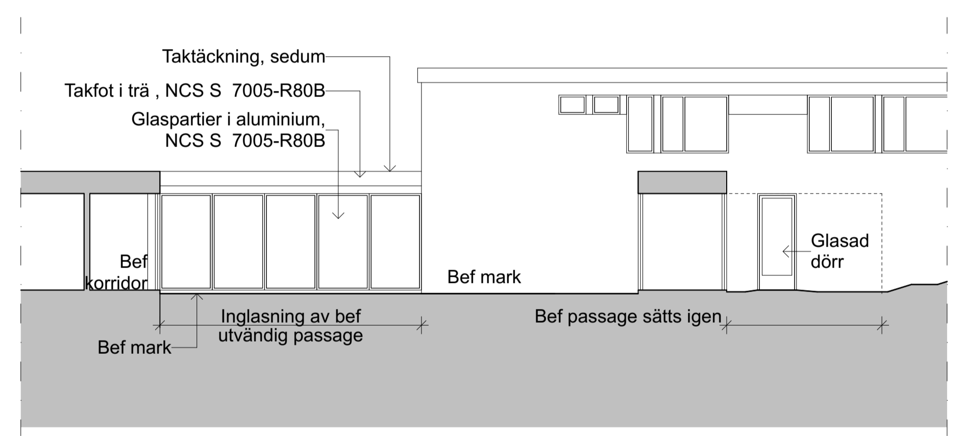
VY 5 Fasad mot öster
