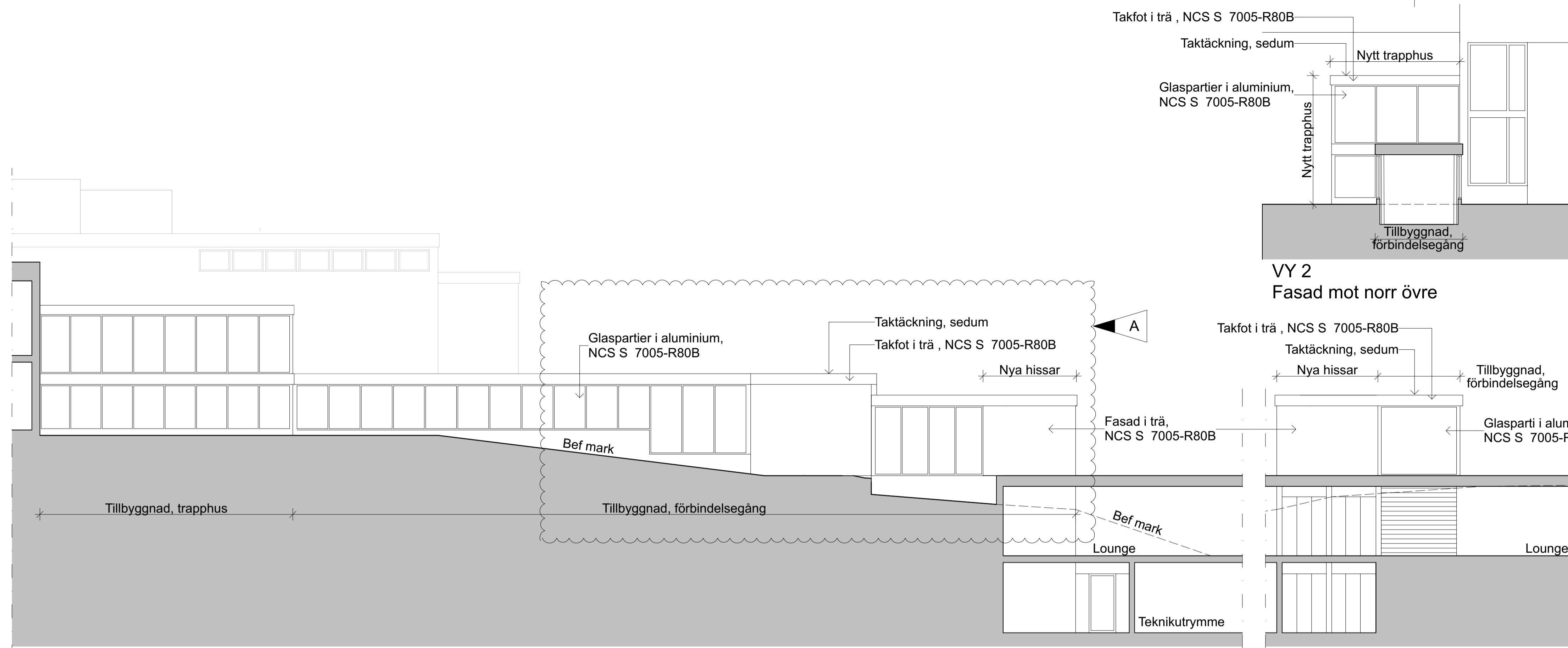
VY 1 FÖRBINDELSEGÅNG MELLAN HUS 1 OCH 3 Fasad mot öster
