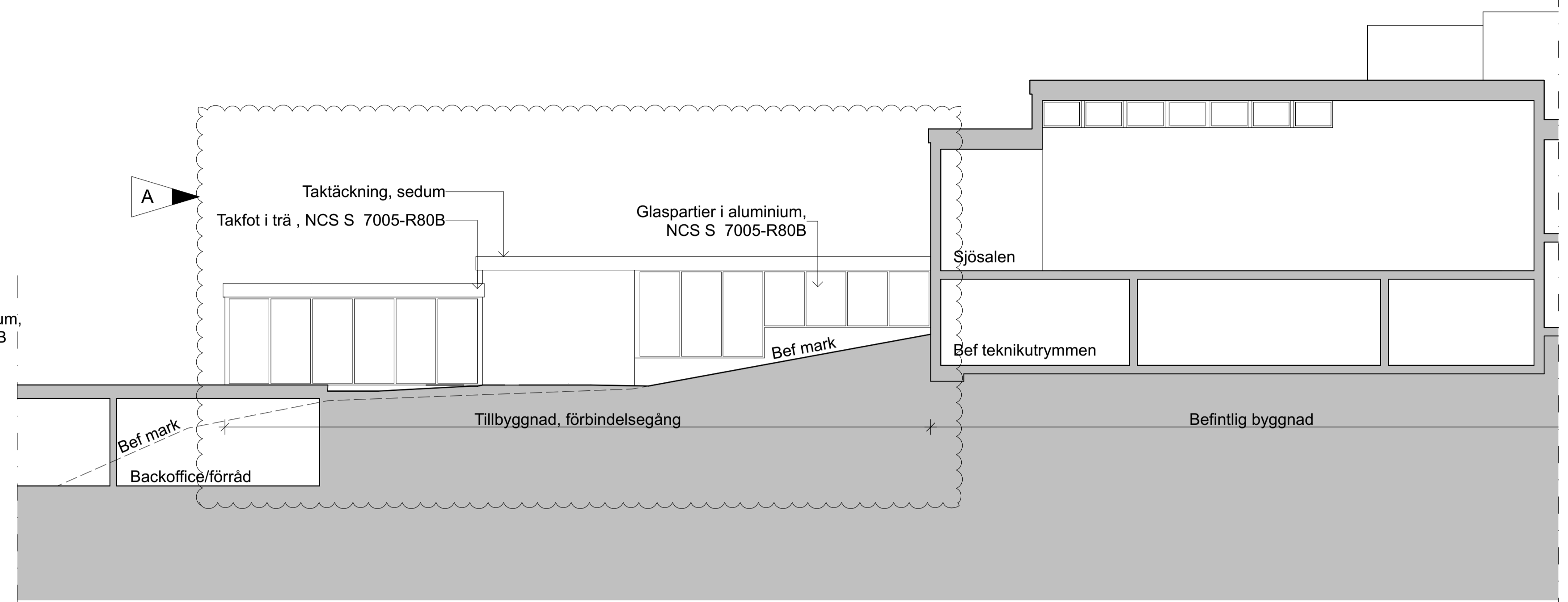
VY 3 Fasad mot norr nedre
