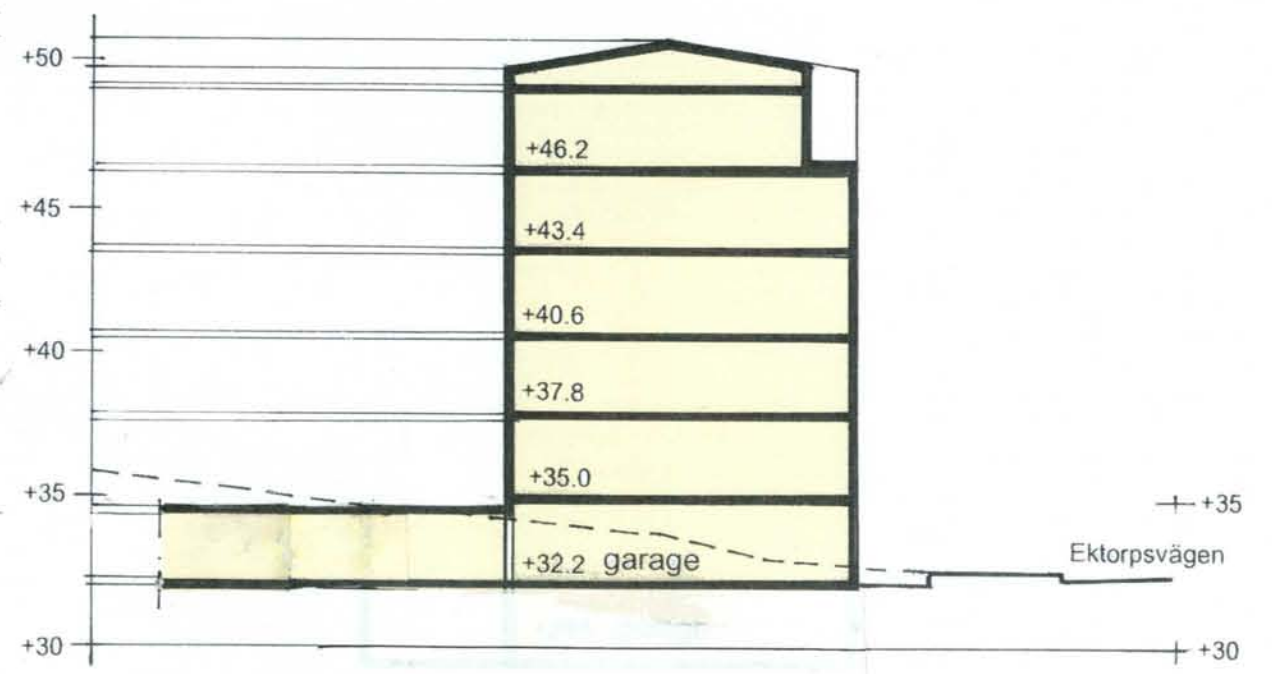
Sektion B-B
