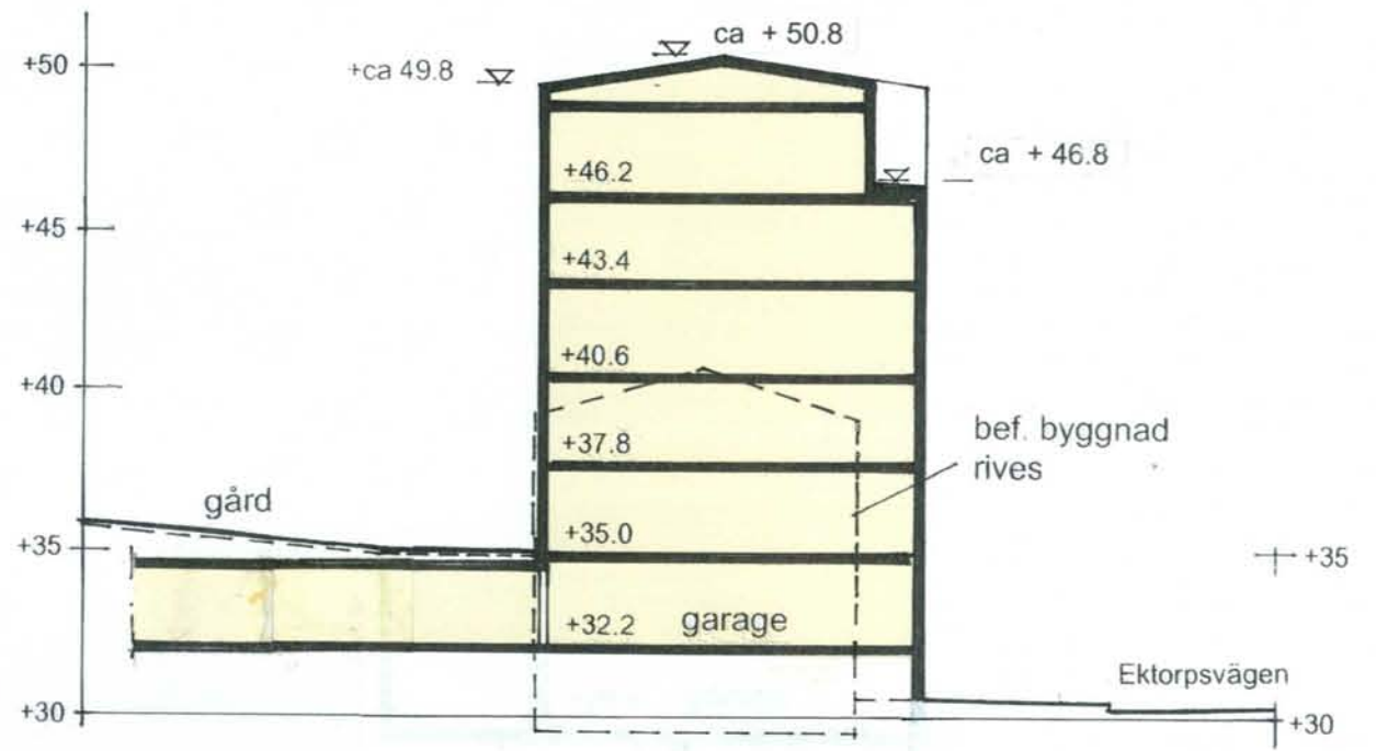
Sektion A-A 1:250
