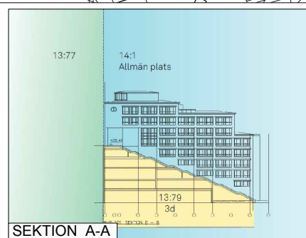
SEKTION A-A
