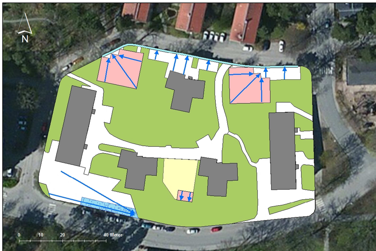
Figur 5-1. Principskiss med ungefärliga placeringar av föreslagen dagvattenhantering. Blå pilar visar hur dagvatten leds på tillkommande hårdgjorda ytor. Ljusblå ytor symboliserar ungefärlig placering av infiltrationsstråk och makadammagasin.
