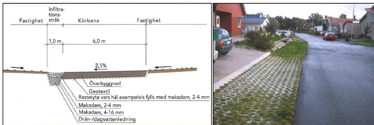
Figur 5-2. Principskiss på en dagvattenlösning med infiltrationsstråk till vänster, och en bild från en praktisk tillämpning av infiltrationsstråk till höger.
