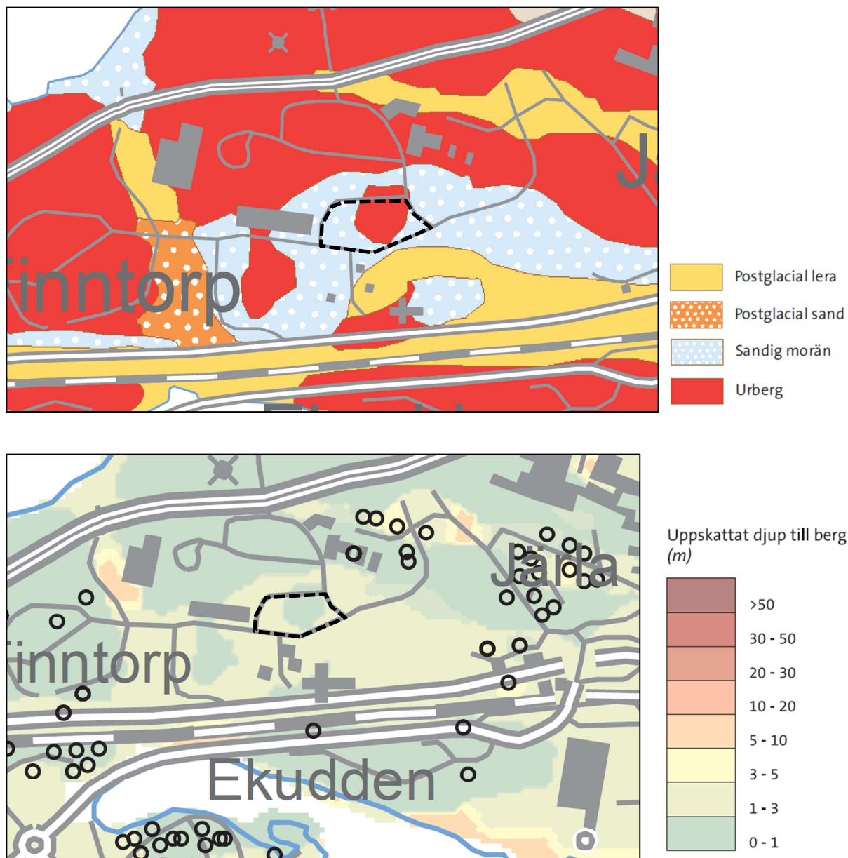
Figur 3-4. Jordartskarta (övre bilden) och jorddjupskarta (nedre bilden) framtagna med SGUs kartgenerator. Svartstreckade polygoner visar den ungefärliga placeringen av fastigheten Sicklaön 125:3.
