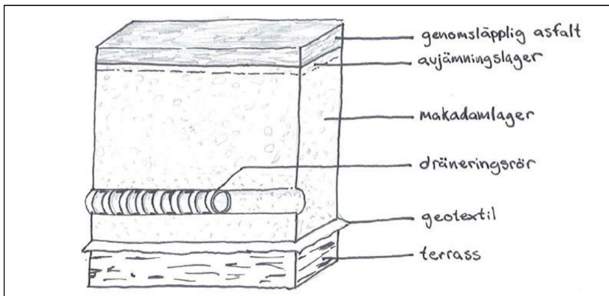
Figur 5-3. Illustration av hur en underbyggnad till en genomsläpplig asfalt kan byggas upp (Bäckström, 1998).
